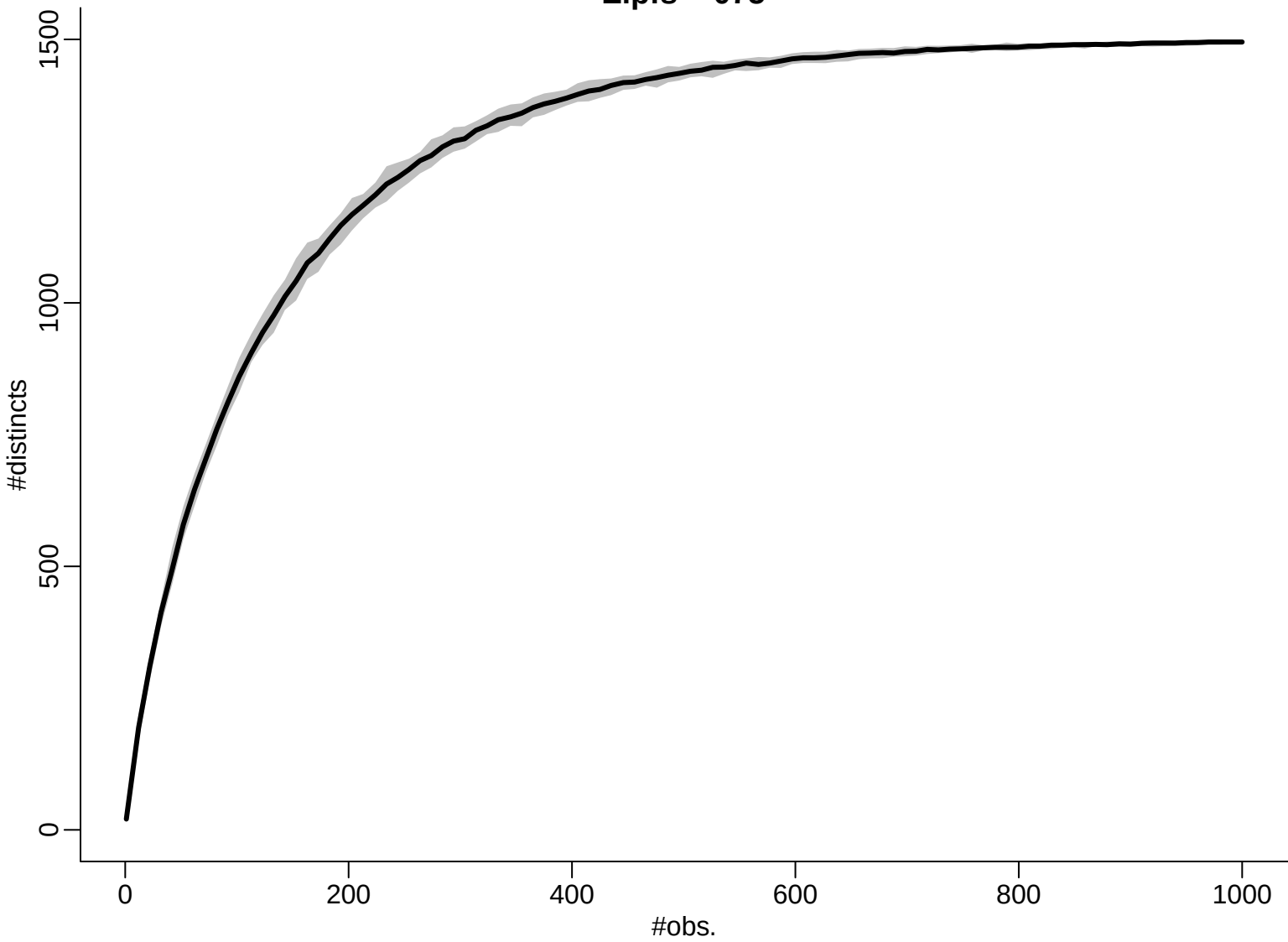
Zipfs - 075
