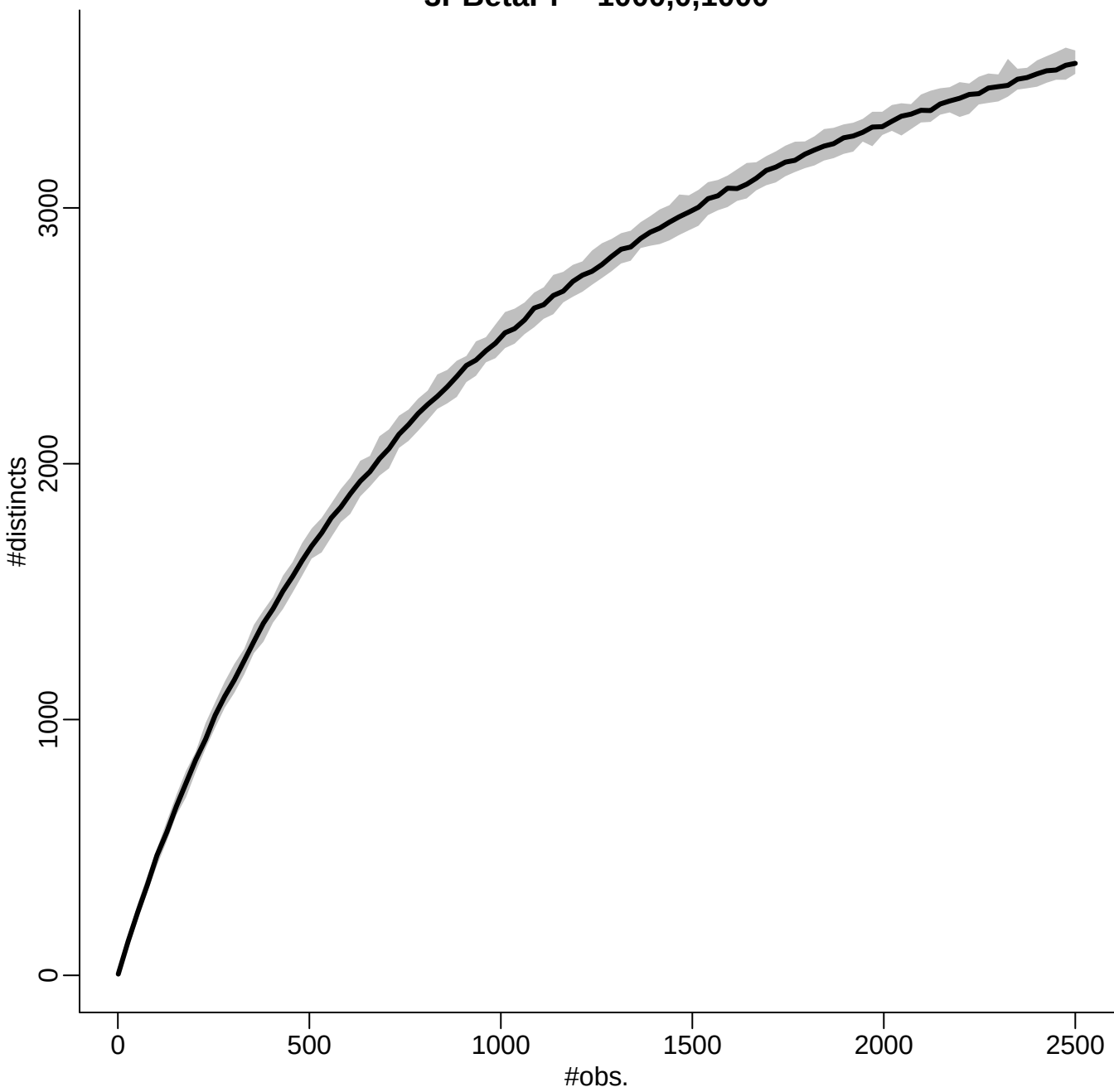
3PBetaPr - 1000,0,1000
