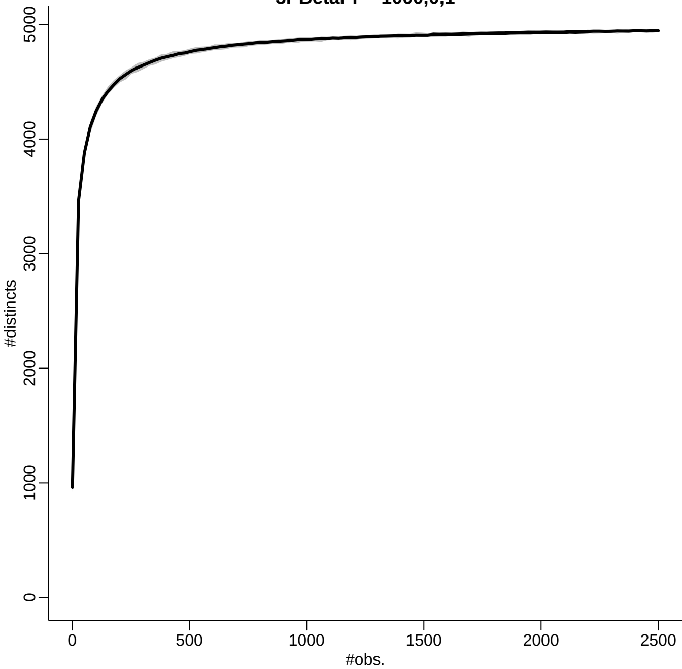
3PBetaPr - 1000,0,1
