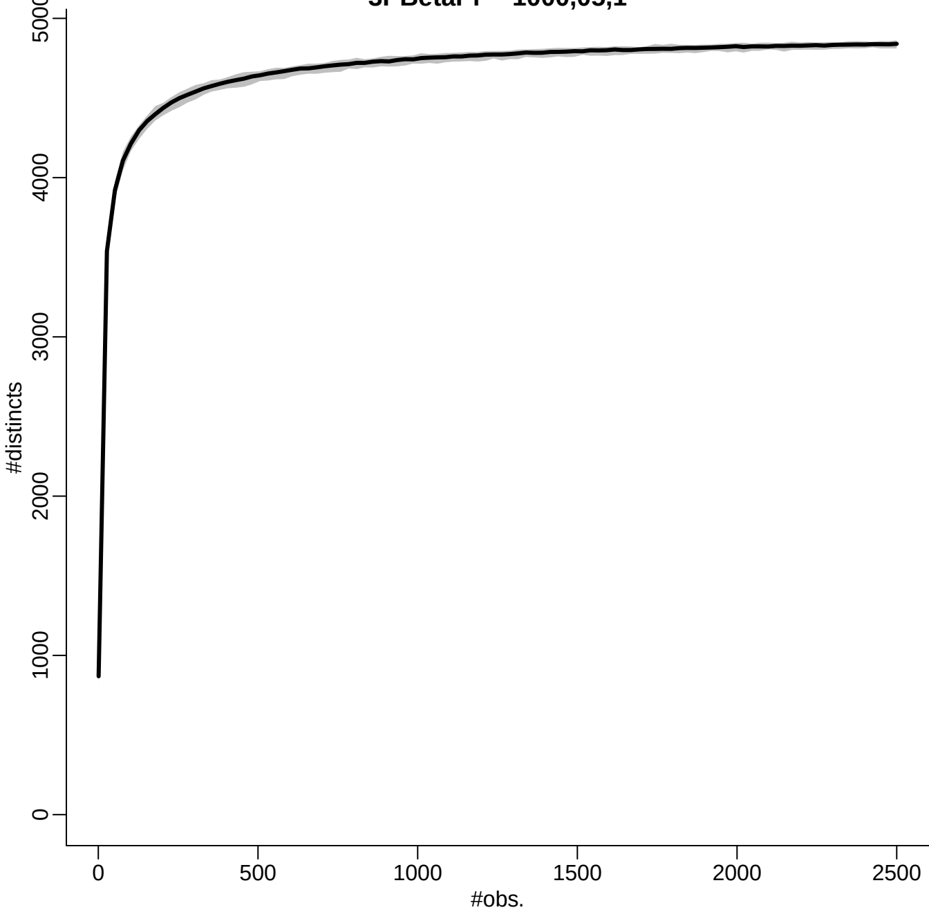
3PBetaPr - 1000,05,1
