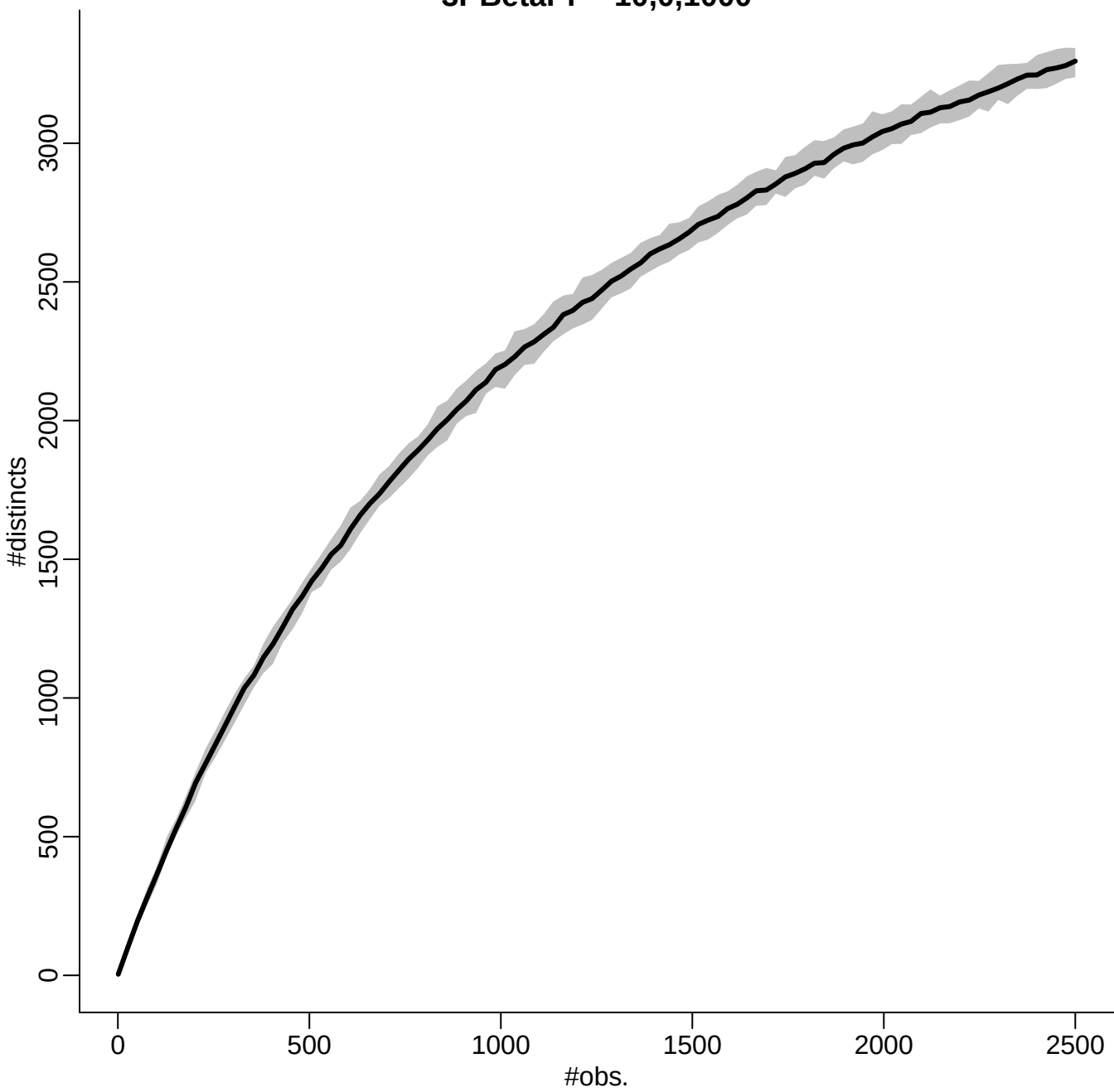
3PBetaPr - 10,0,1000
