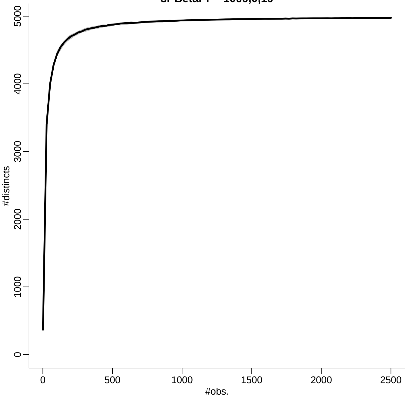
3PBetaPr - 1000,0,10
