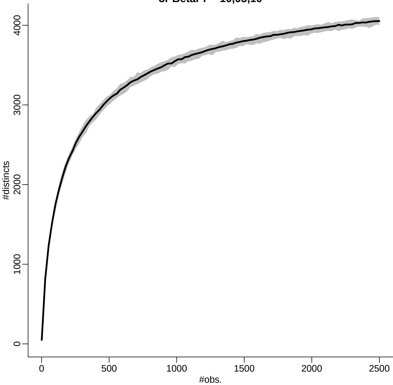
3PBetaPr – 10,05,10
