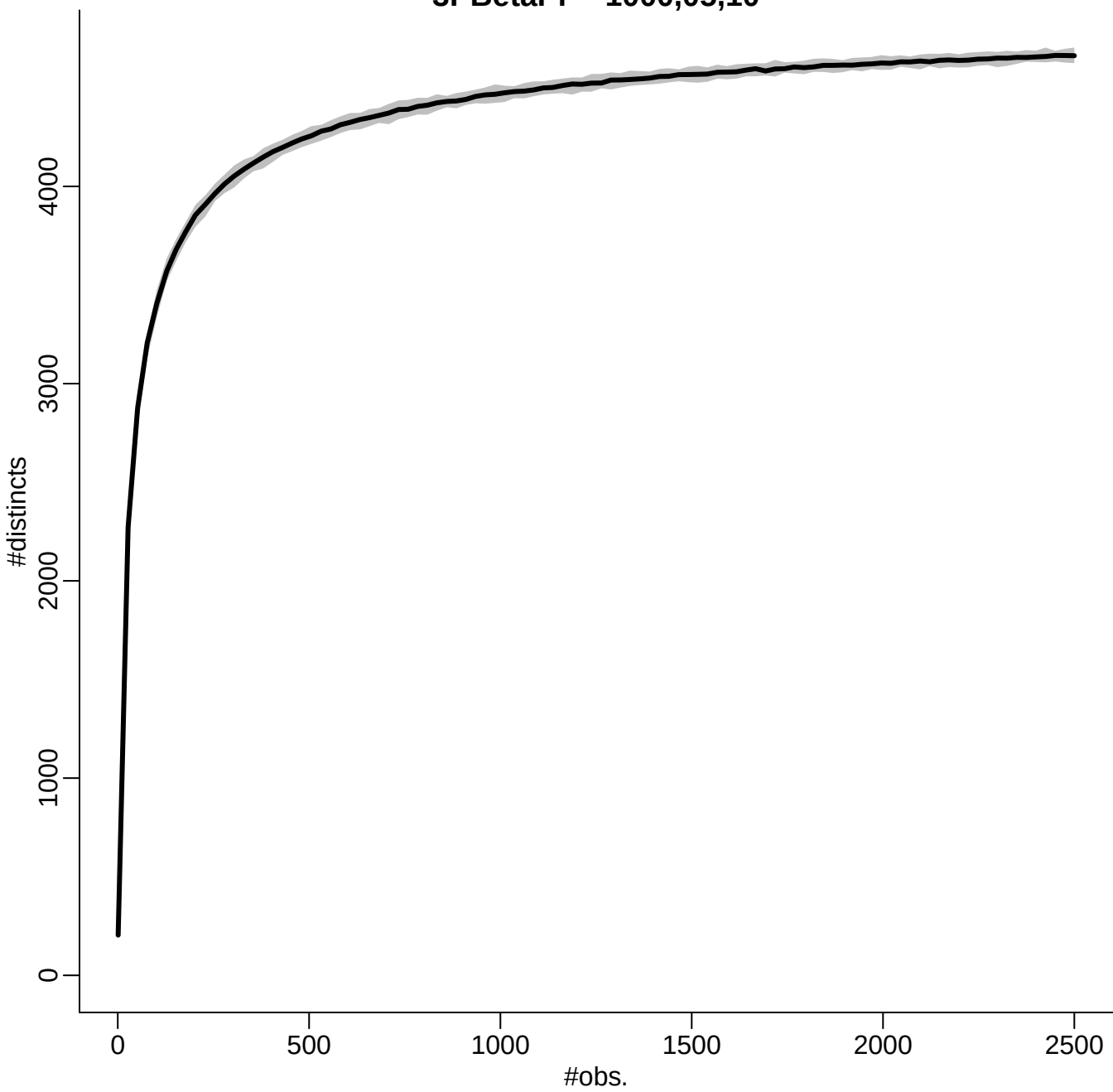
3PBetaPr – 1000,05,10
