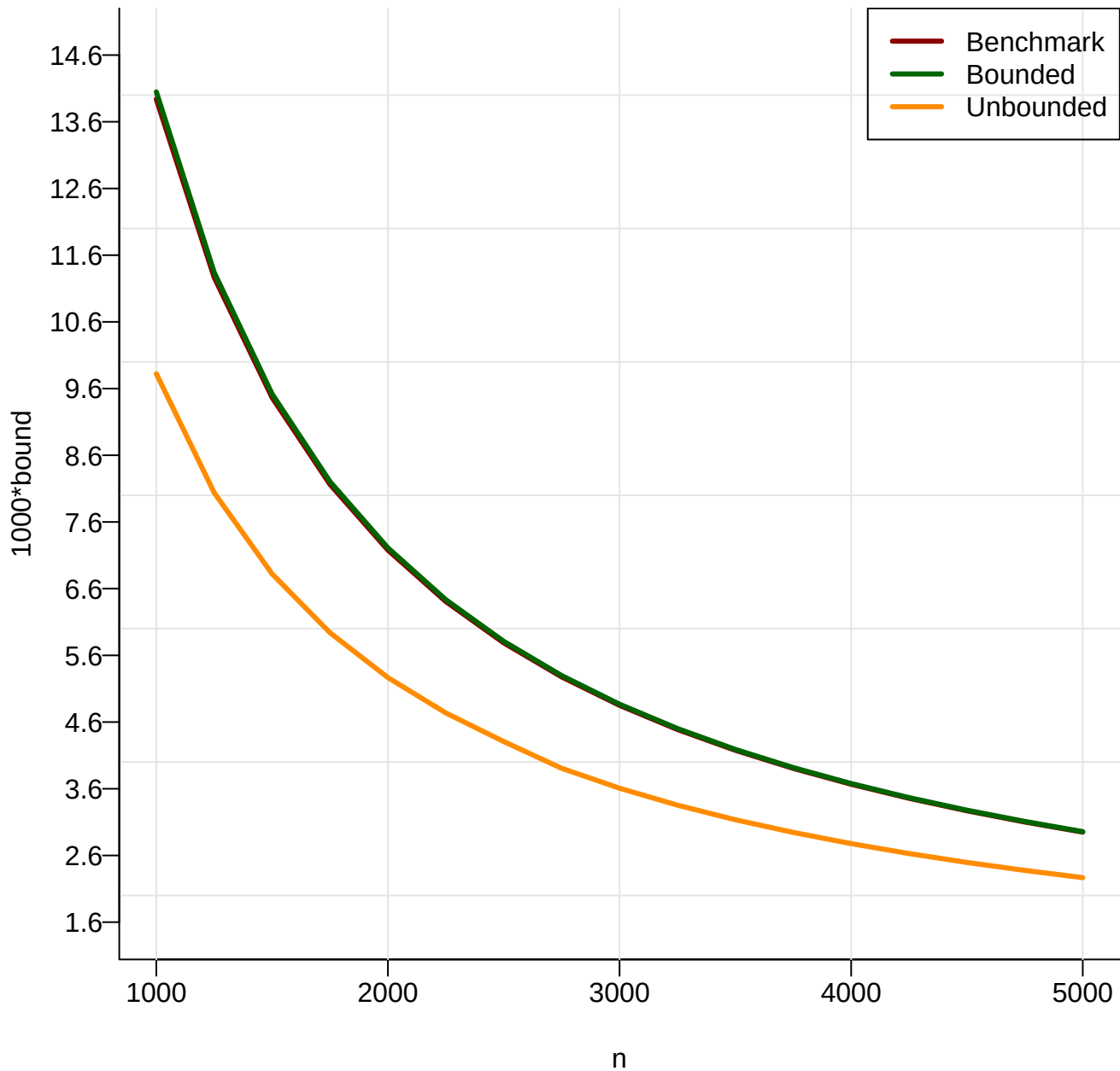
3PBetaPr – 10,0,1000
