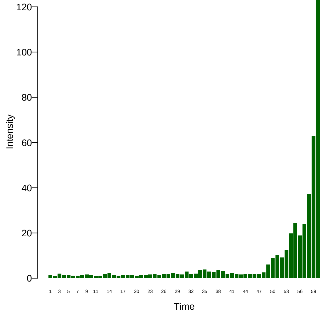
Xi: 22
