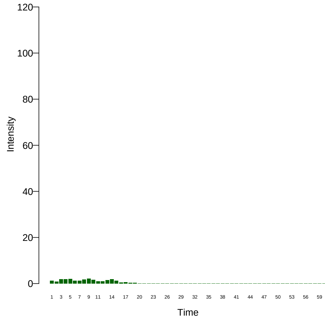
Xi: 15
