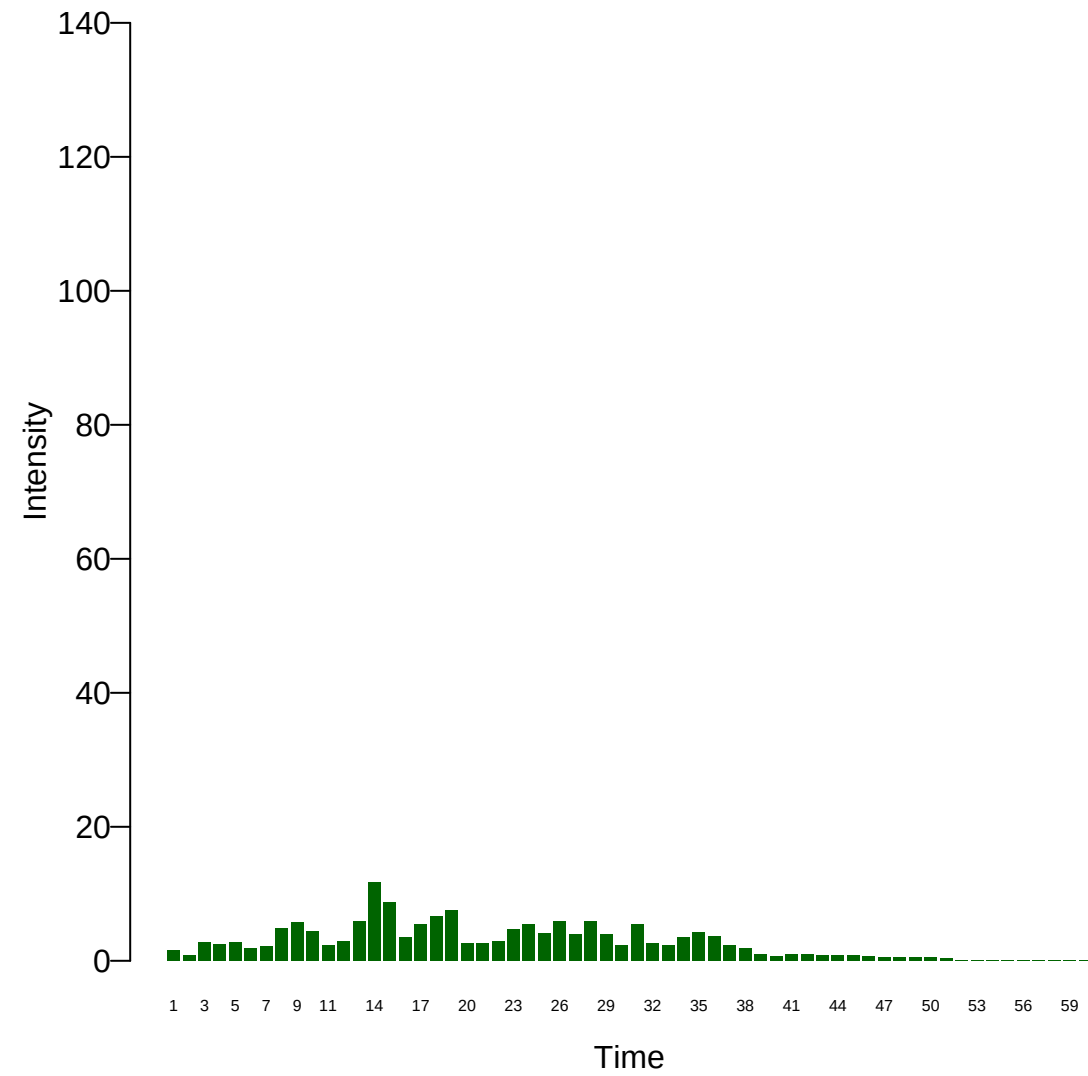
Xi: 39
