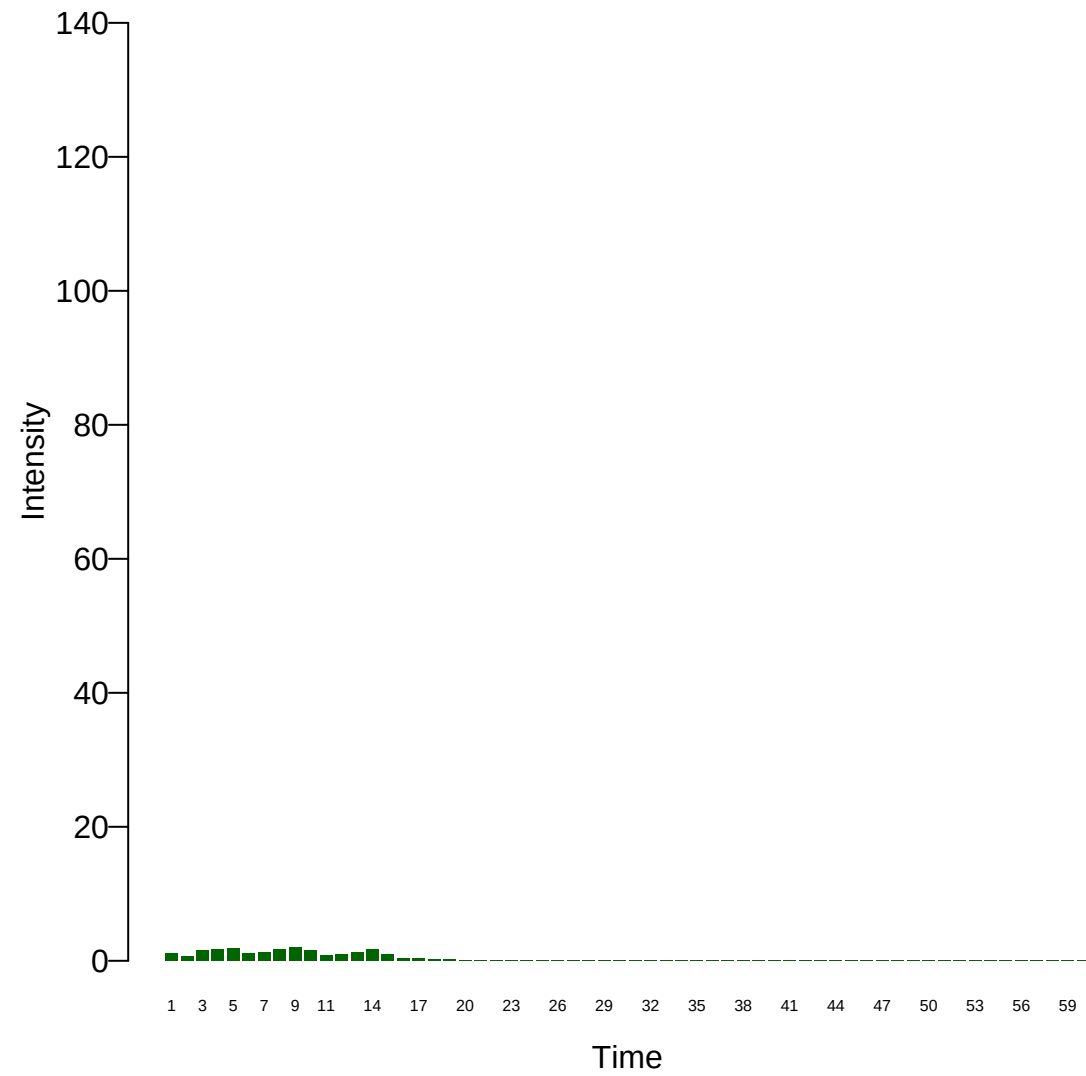
Xi: 24
