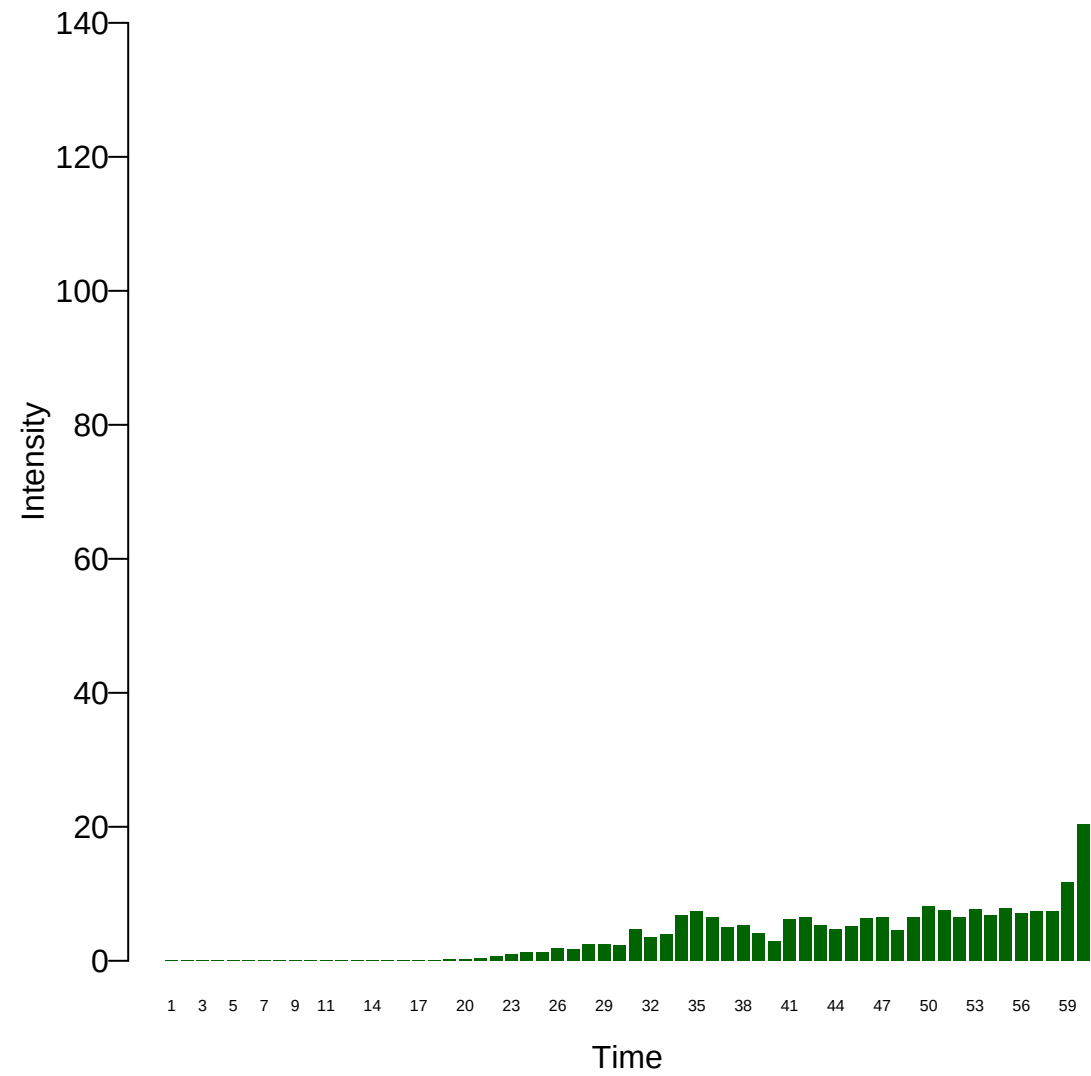
Xi: 19
