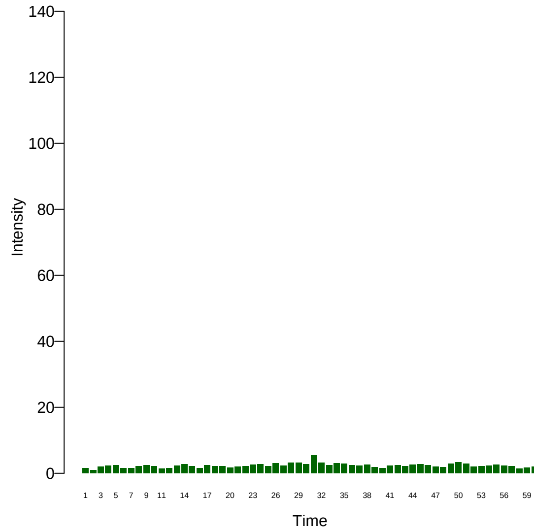
Xi: 5
