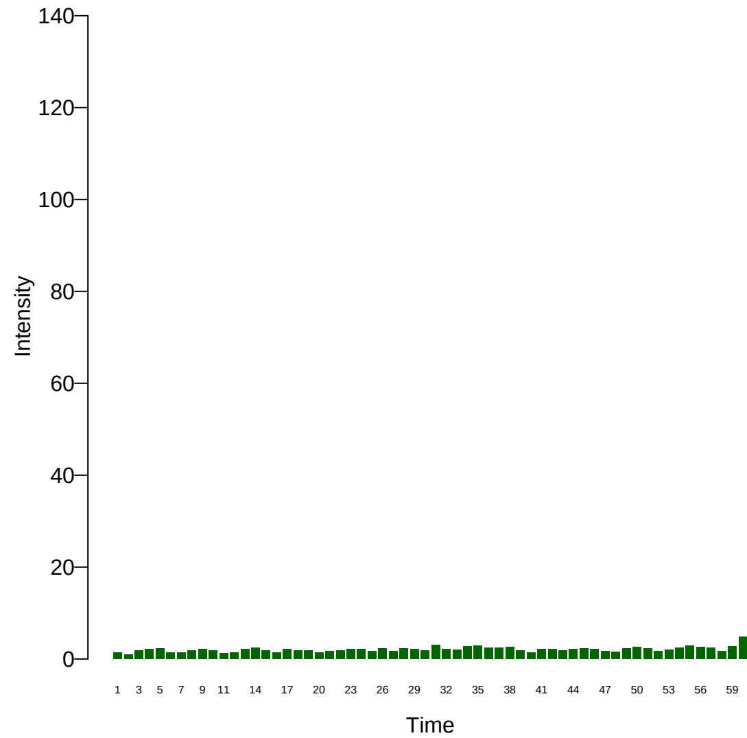
Xi: 10
