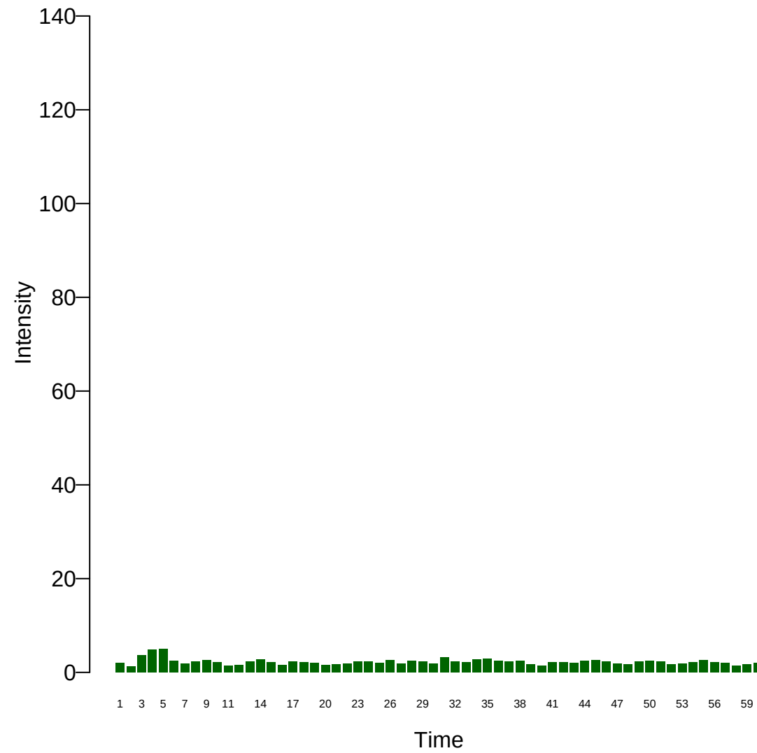
Xi: 6
