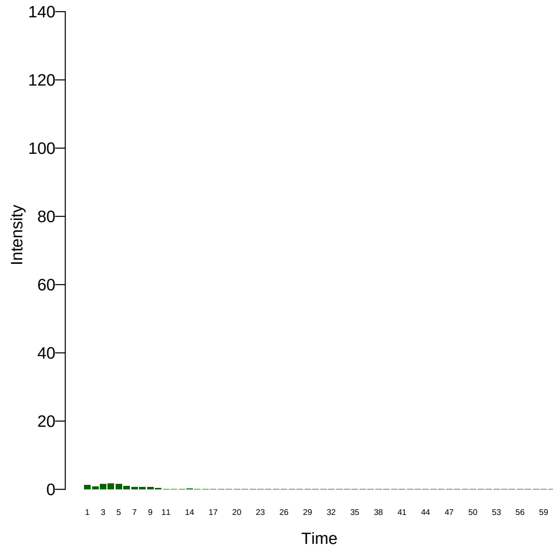
Xi: 22
