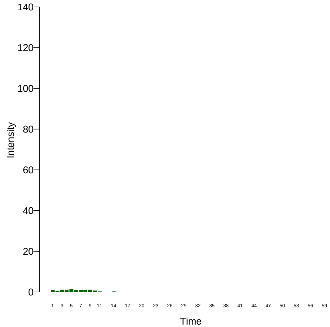
Xi: 36
