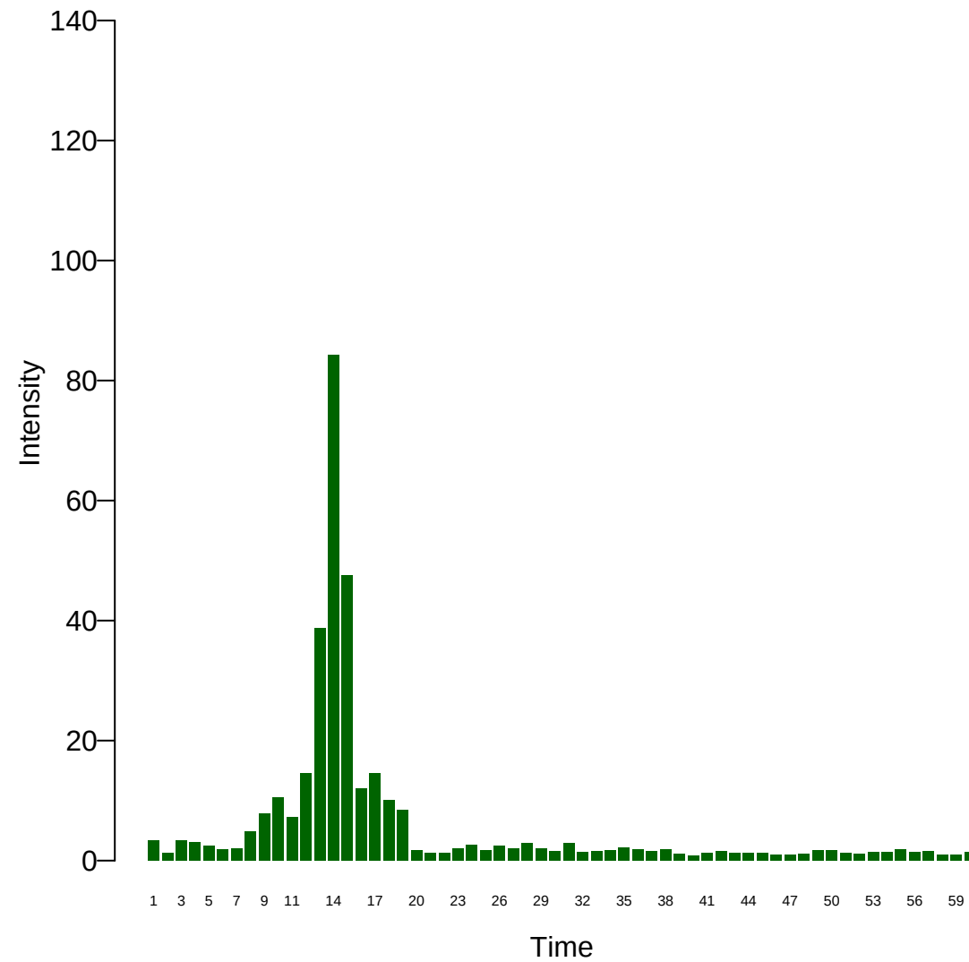
Xi: 28
