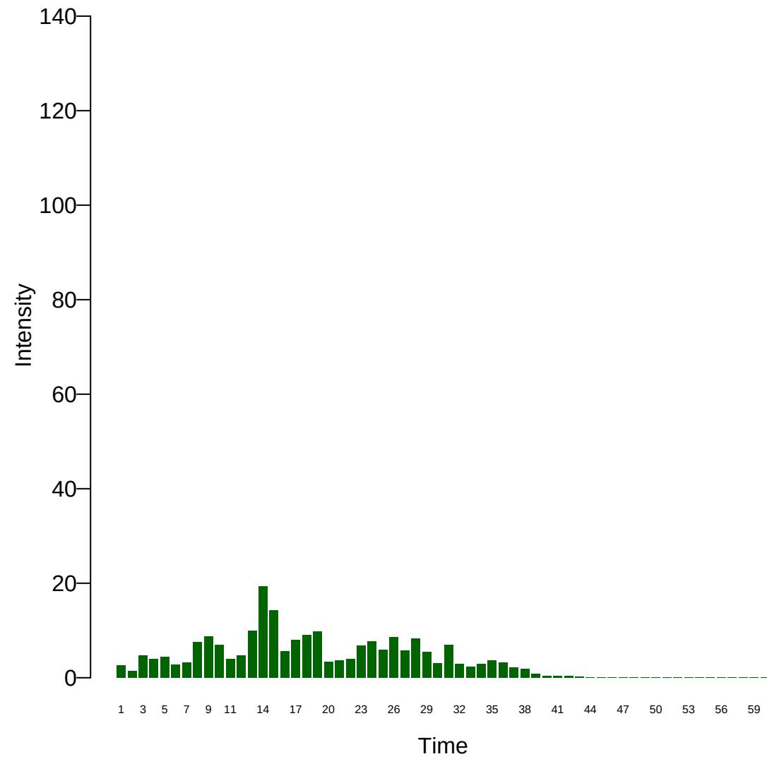
Xi: 27
