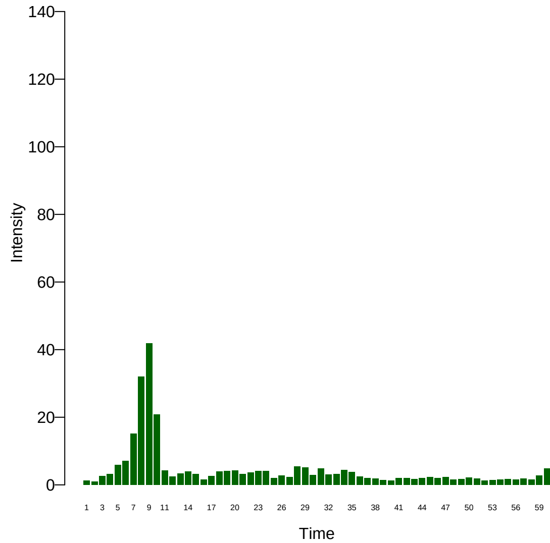
Xi: 13
