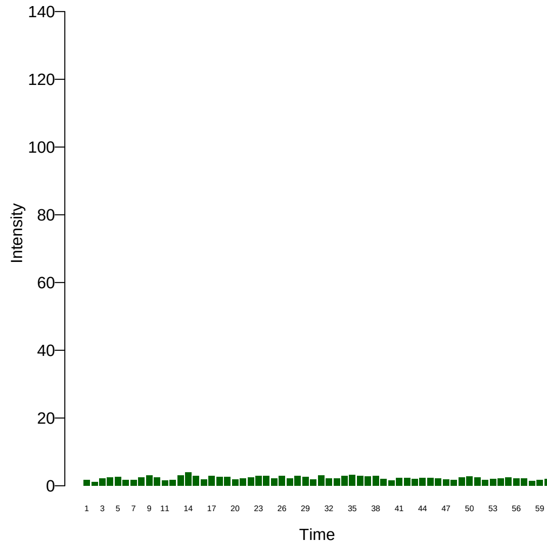
Xi: 4
