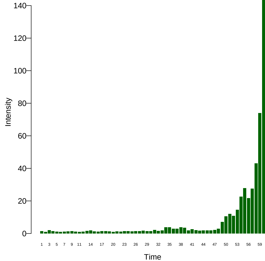
Xi: 20
