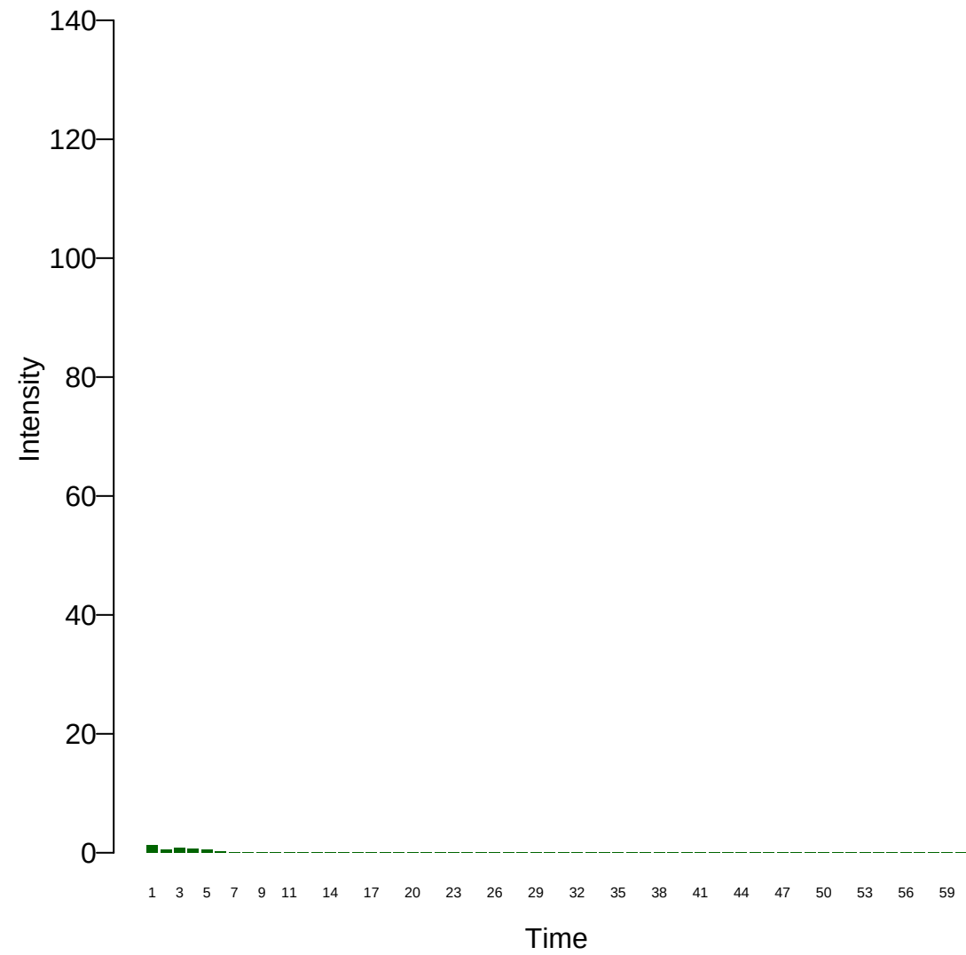
Xi: 17
