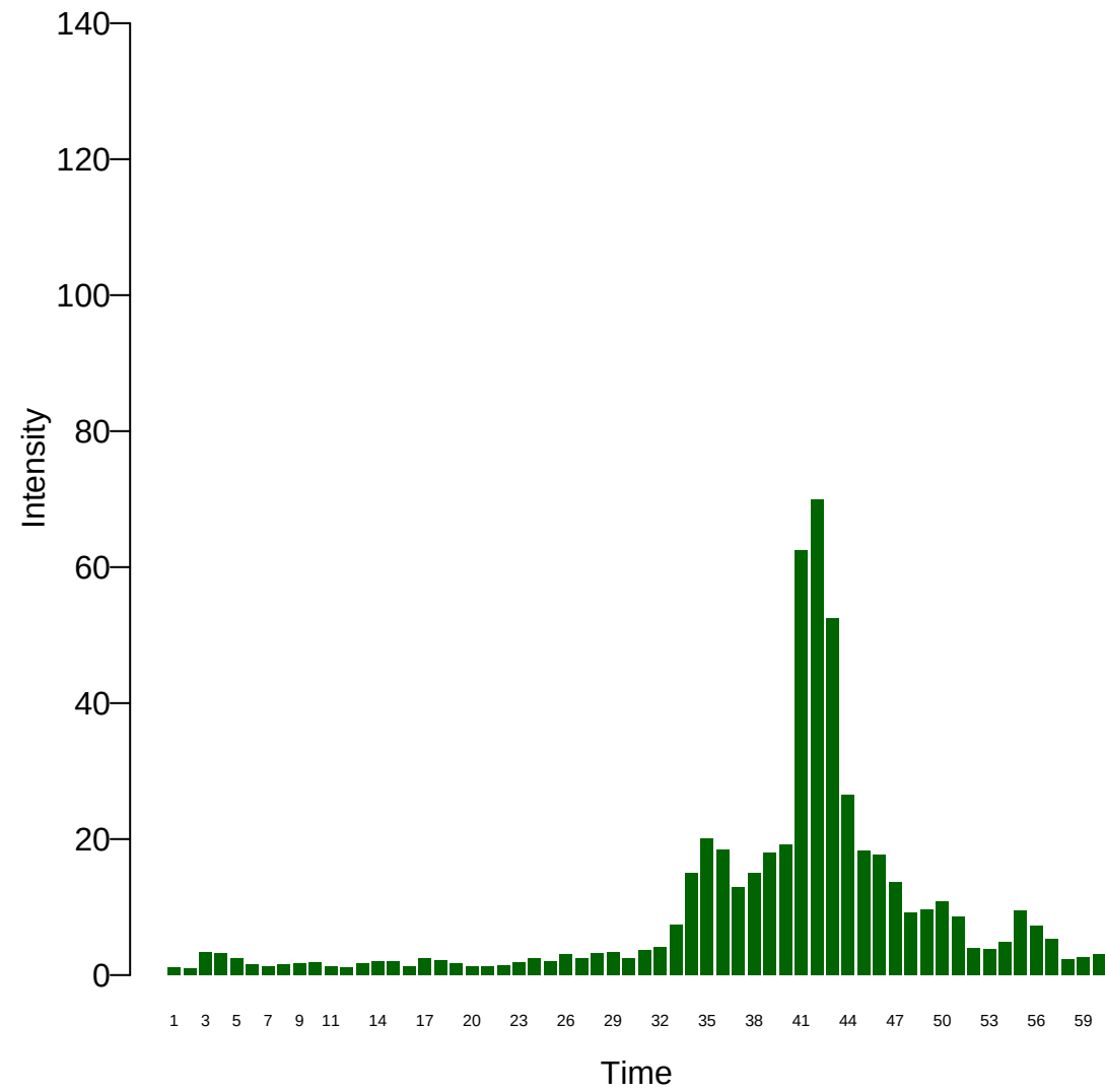
Xi: 16
