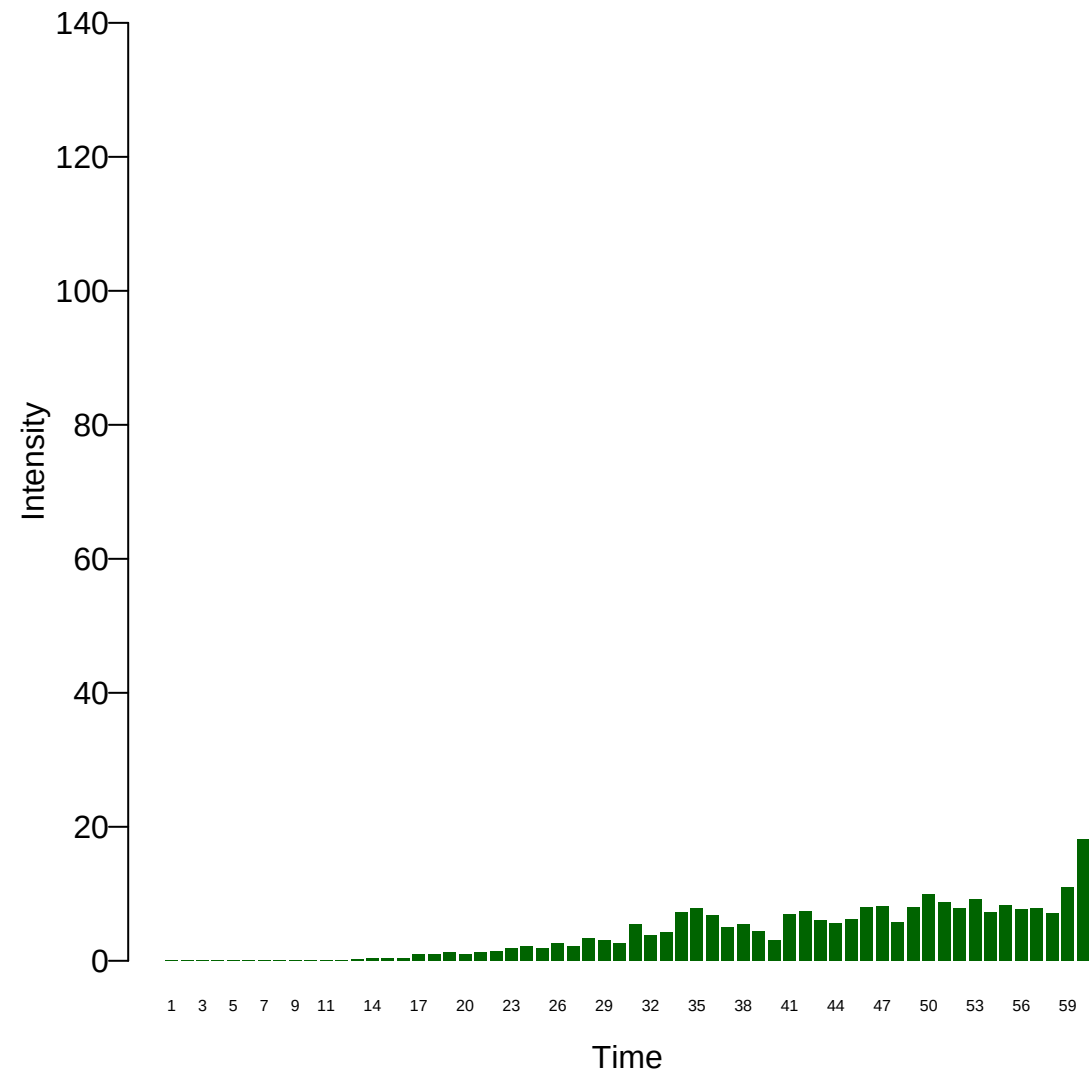
Xi: 23
