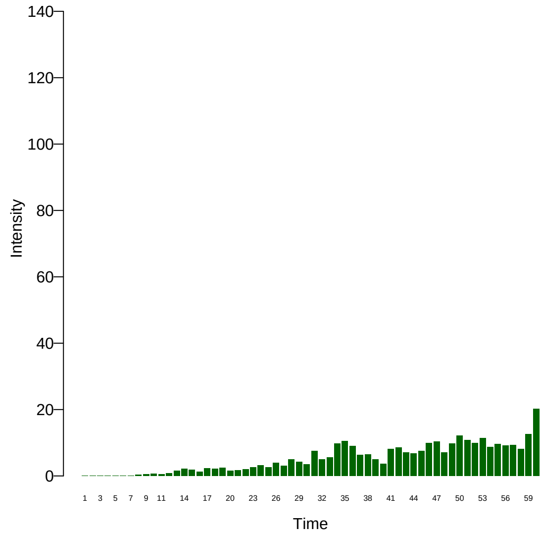
Xi: 12
