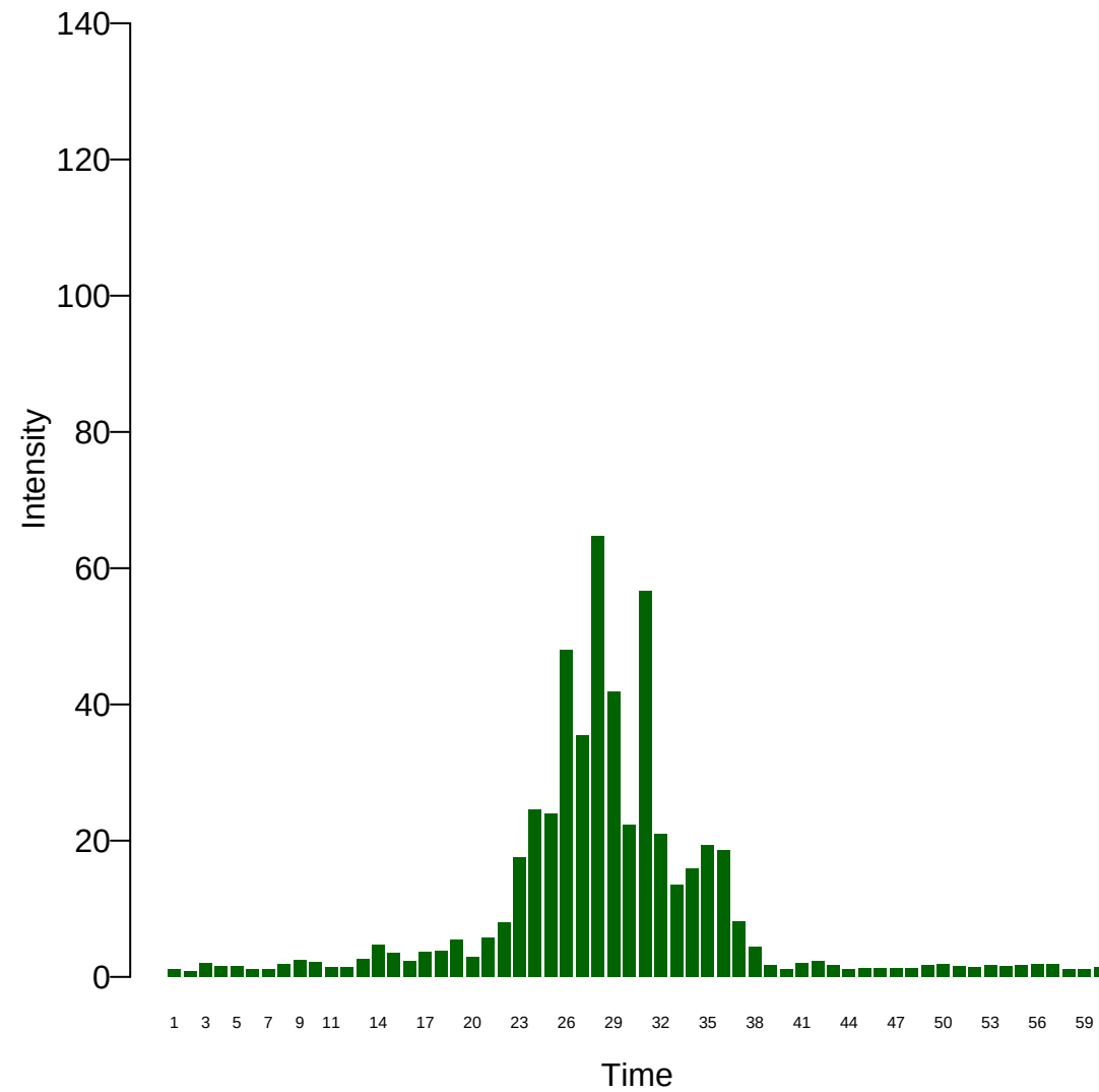
Xi: 15
