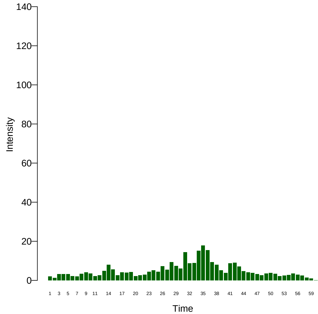
Xi: 2
