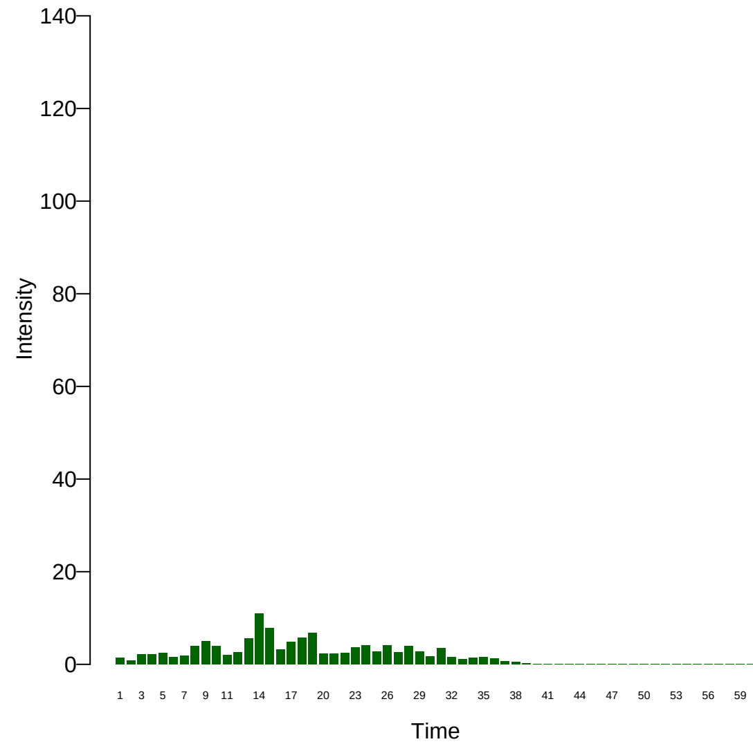
Xi: 32
