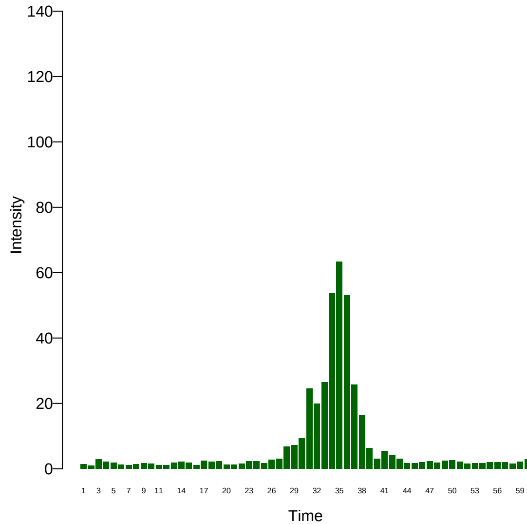
Xi: 25
