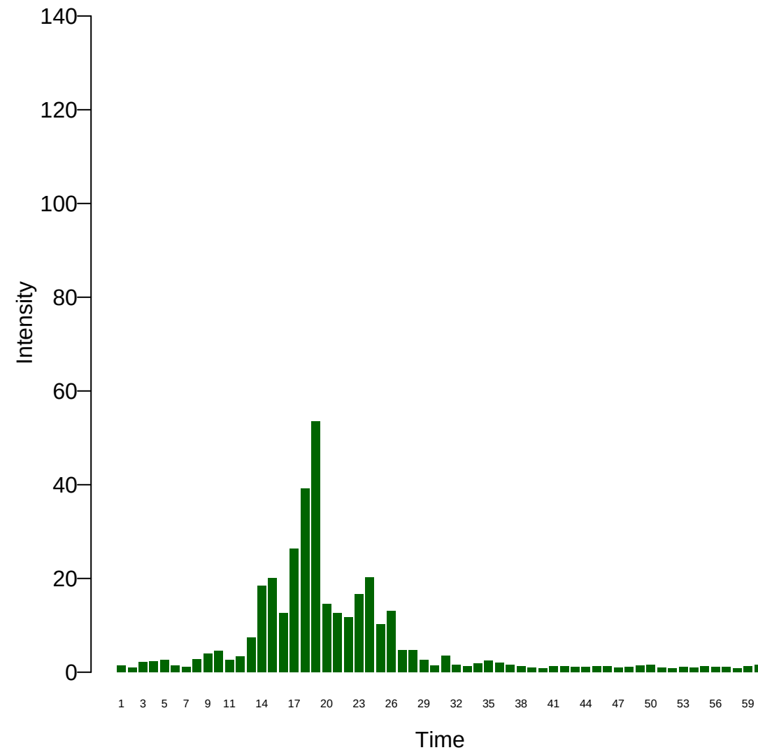
Xi: 31
