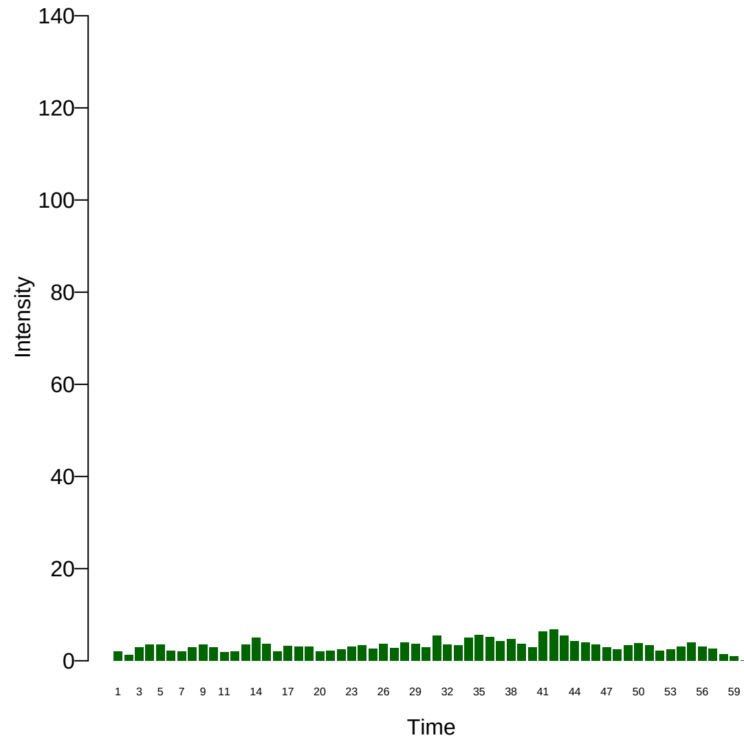
Xi: 1
