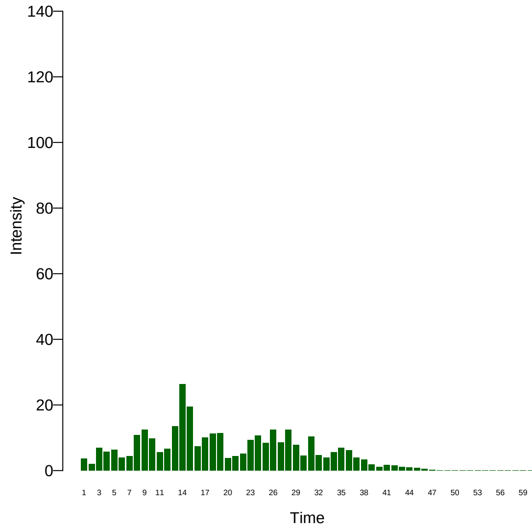
Xi: 21
