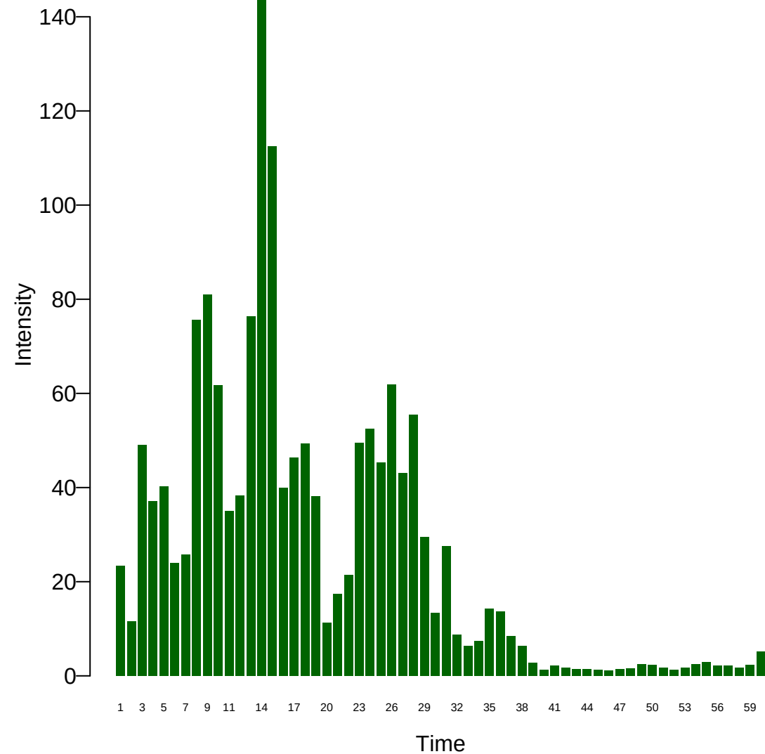
Xi: 11
