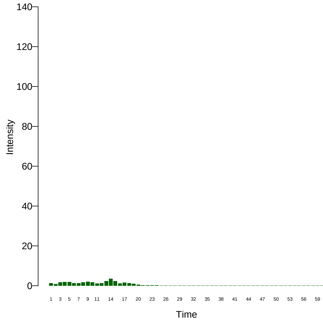
Xi: 18
