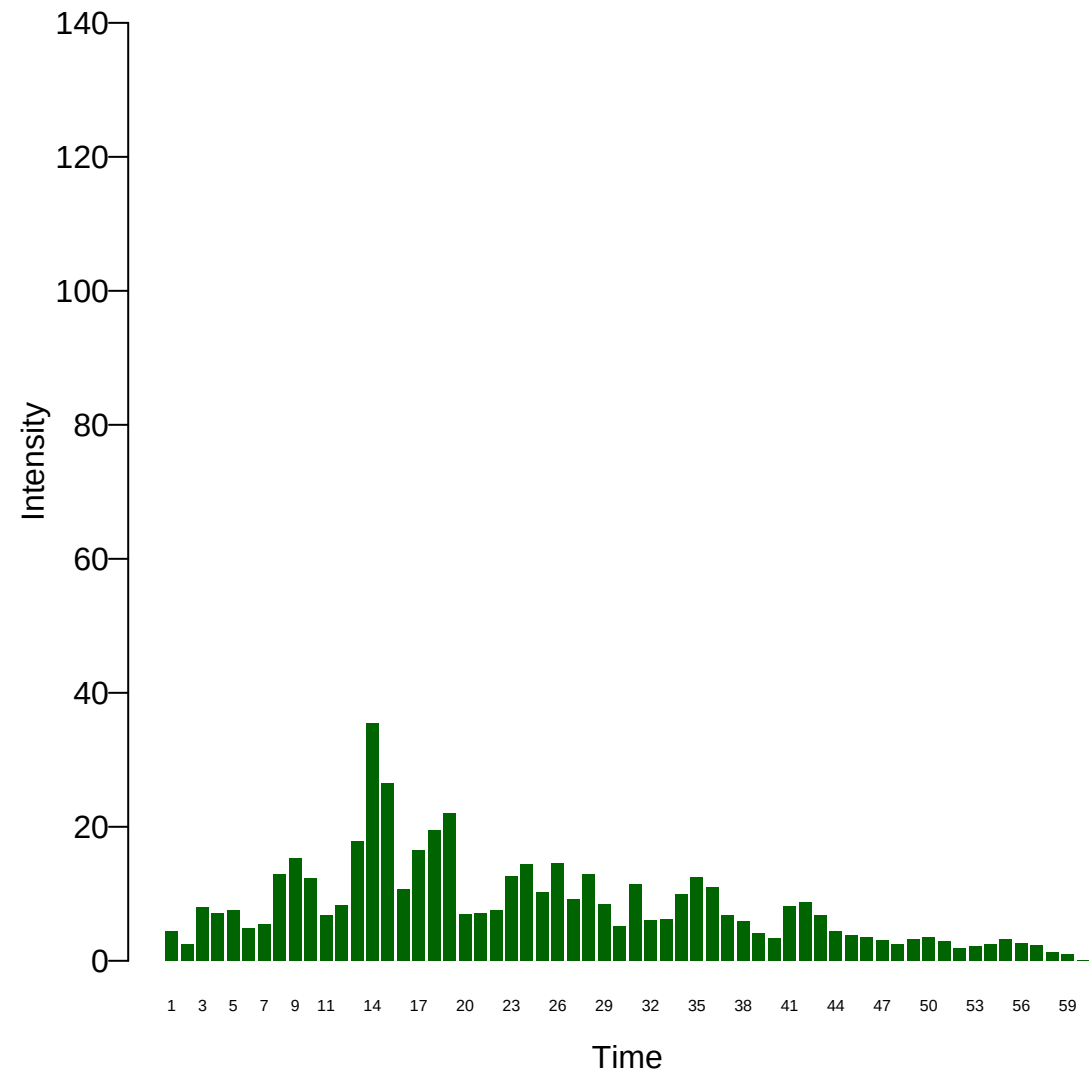
Xi: 3
