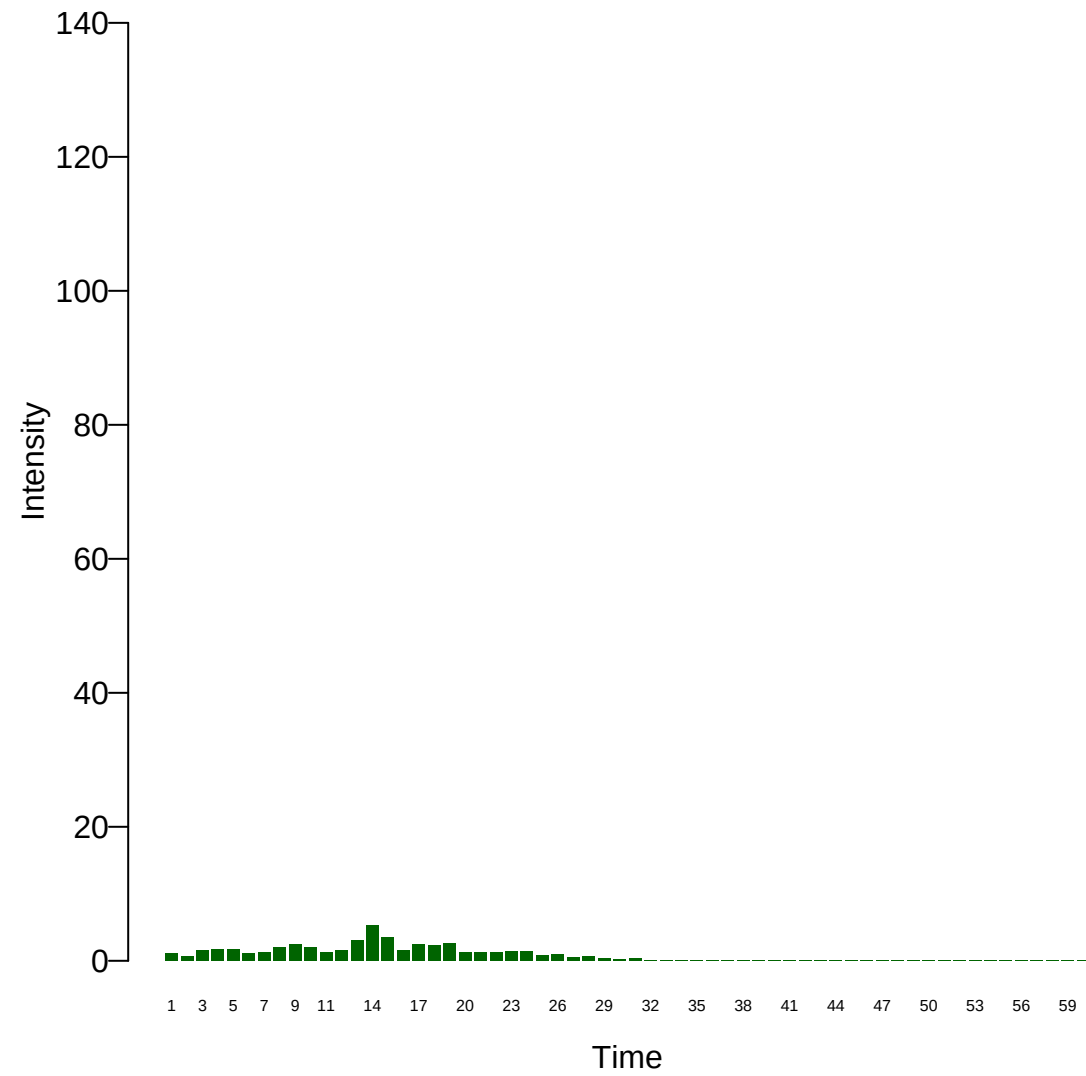
Xi: 26
