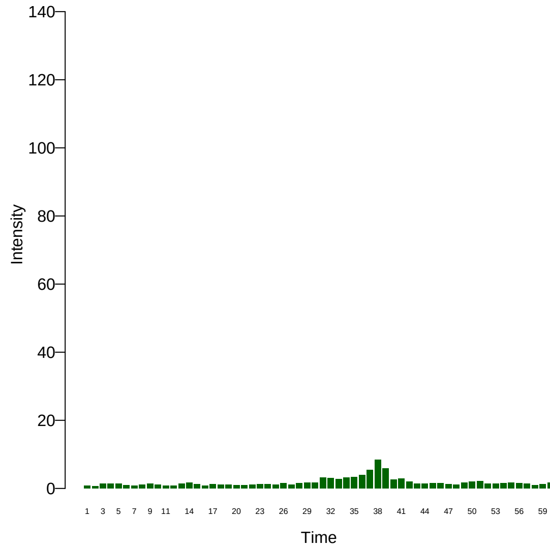
Xi: 33
