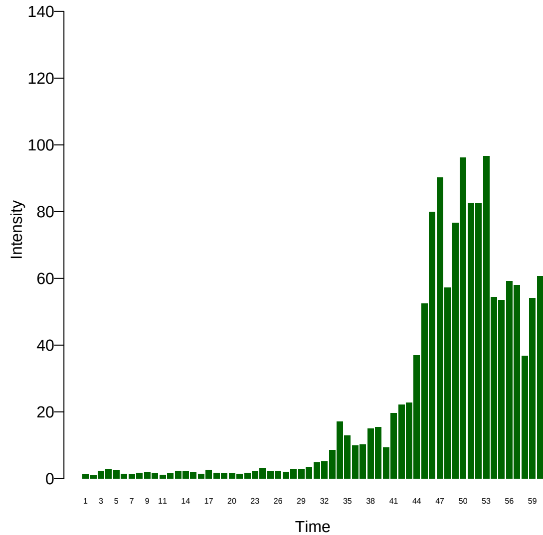
Xi: 7
