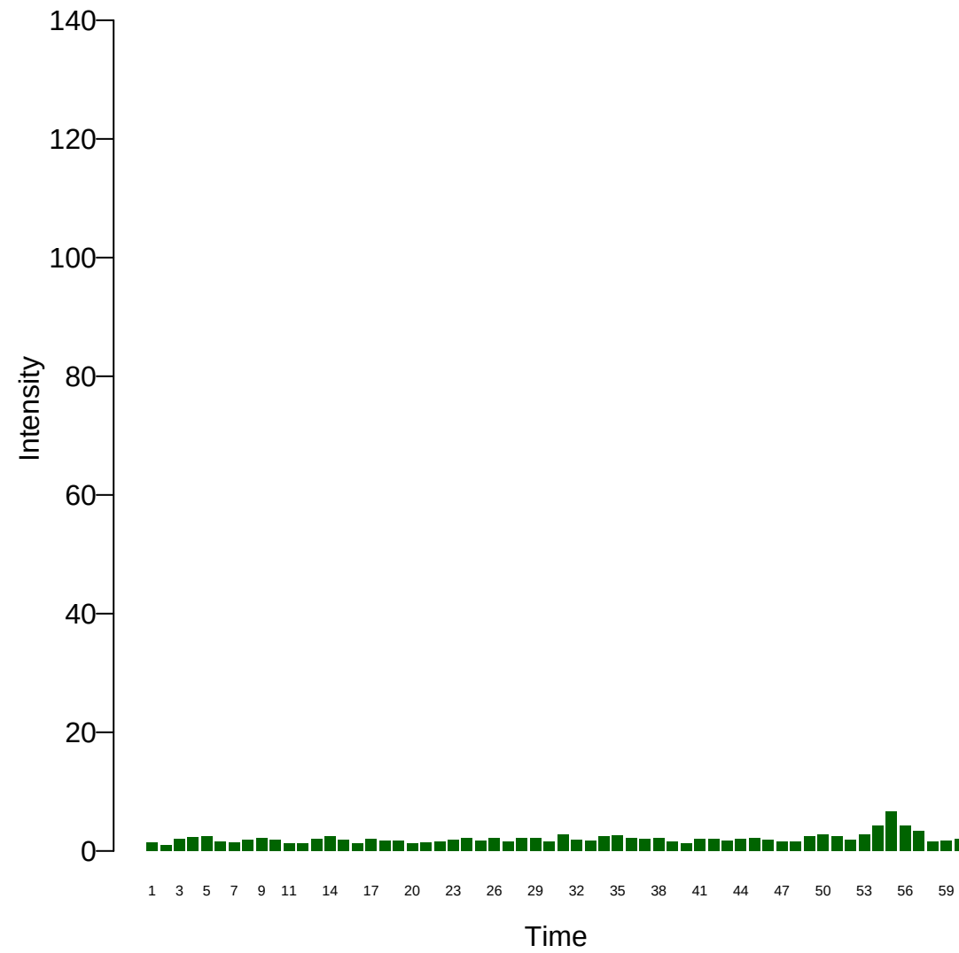
Xi: 14
