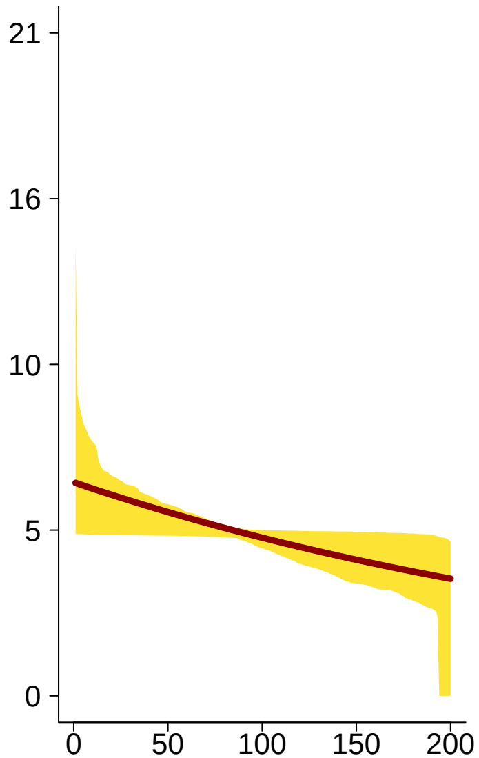
Prob * 1000 (DiriMulti)
