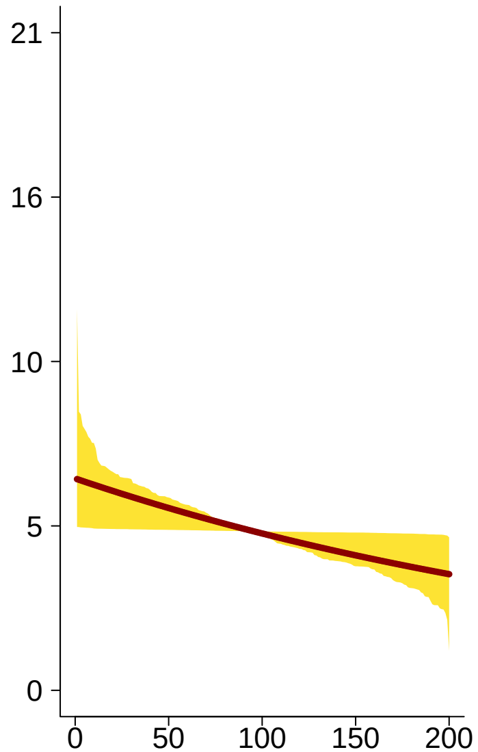
Prob * 1000 (DiriMulti)
