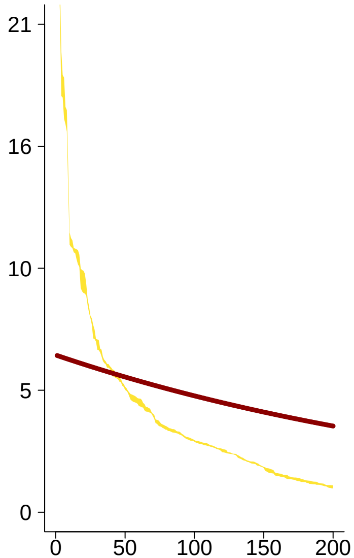
Prob * 1000 (FDP)
