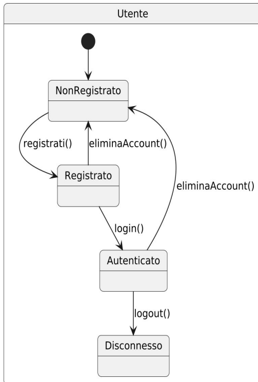
Statechart - Utente
