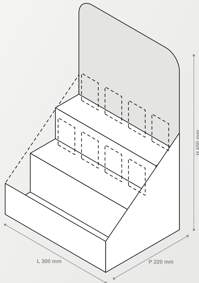
Espositore da banco a gradini — assonometria
