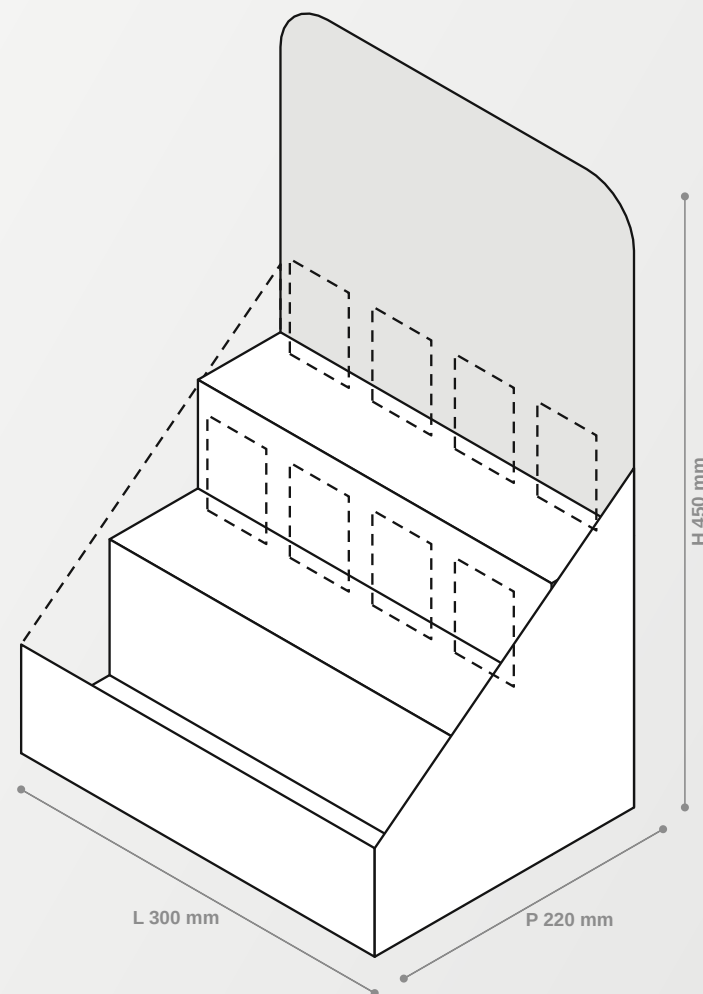
Fig. 03 — Espositore da banco a gradini, quote indicative
