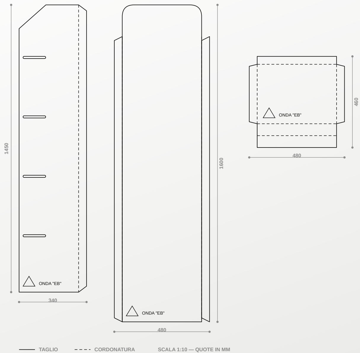
Fig. 05 — Fianco, schienale e ripiano, scala 1:10
