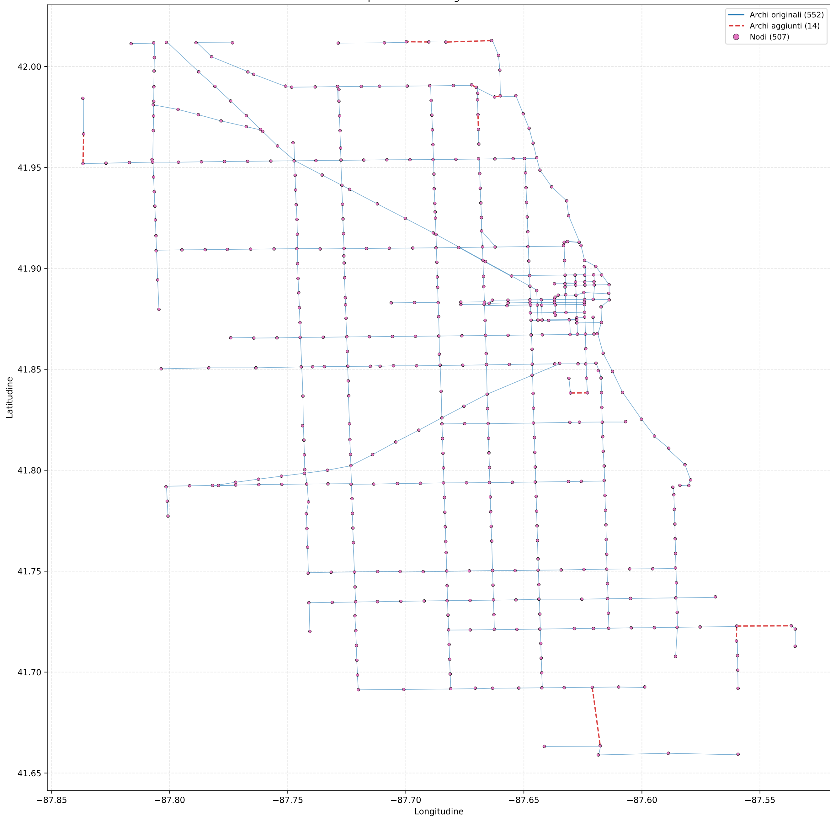
Grafo processato Chicago — archi e nodi
