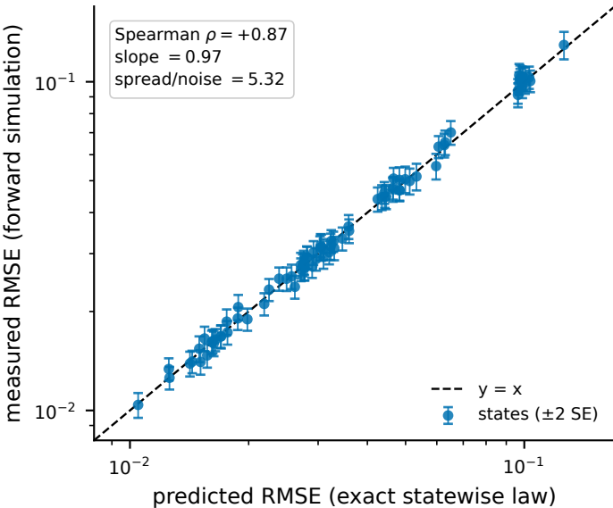
varying estimand (variable-rank Ginibre)
