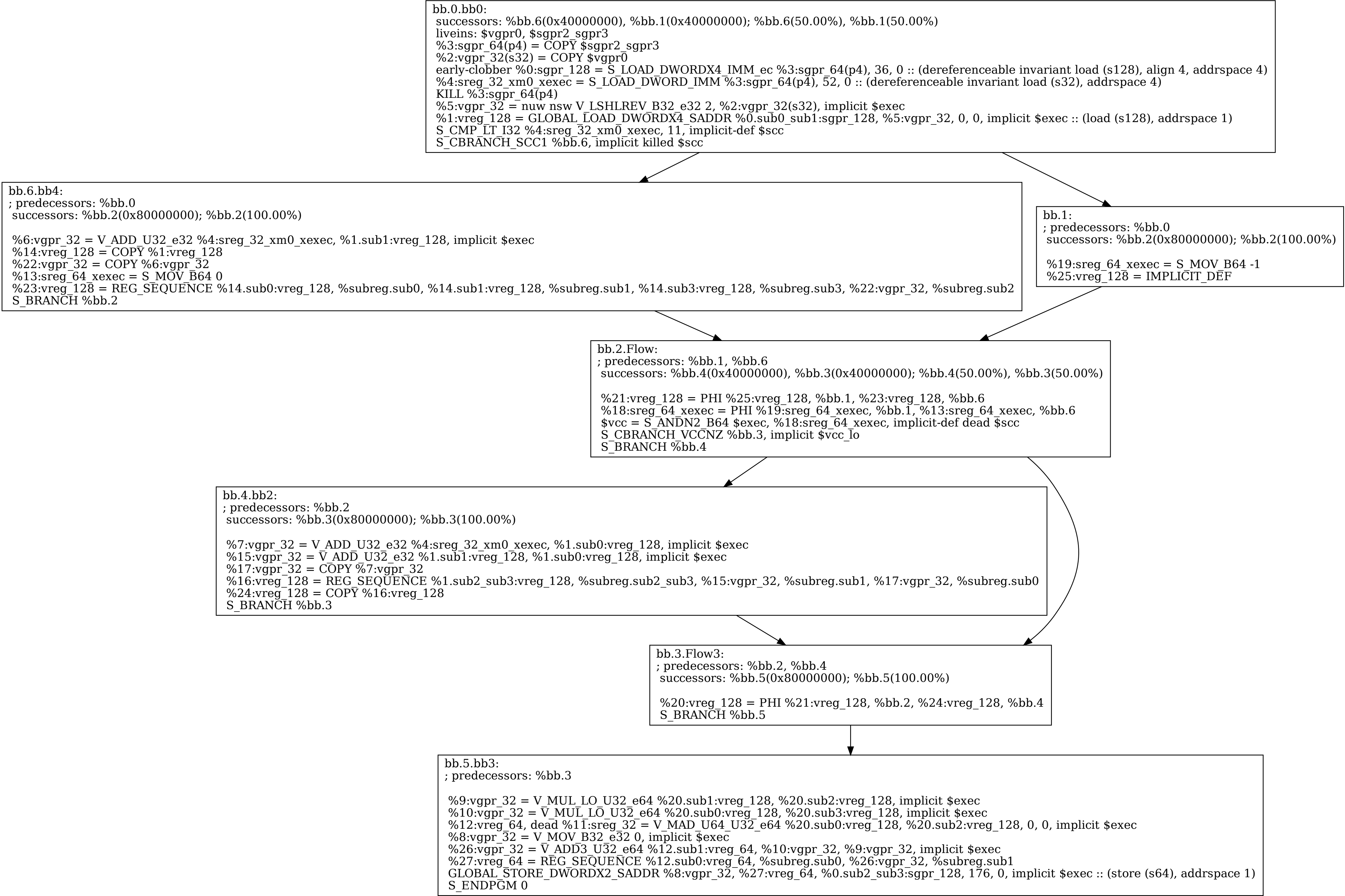
CFG for 'test_subregs' function
