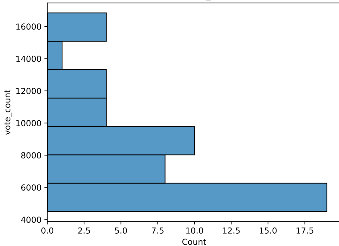
Гистограмма vote_count (Excel)
