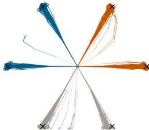
IMLE
