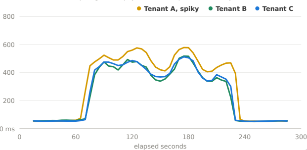
Rolling p50 TTFT per tenant
