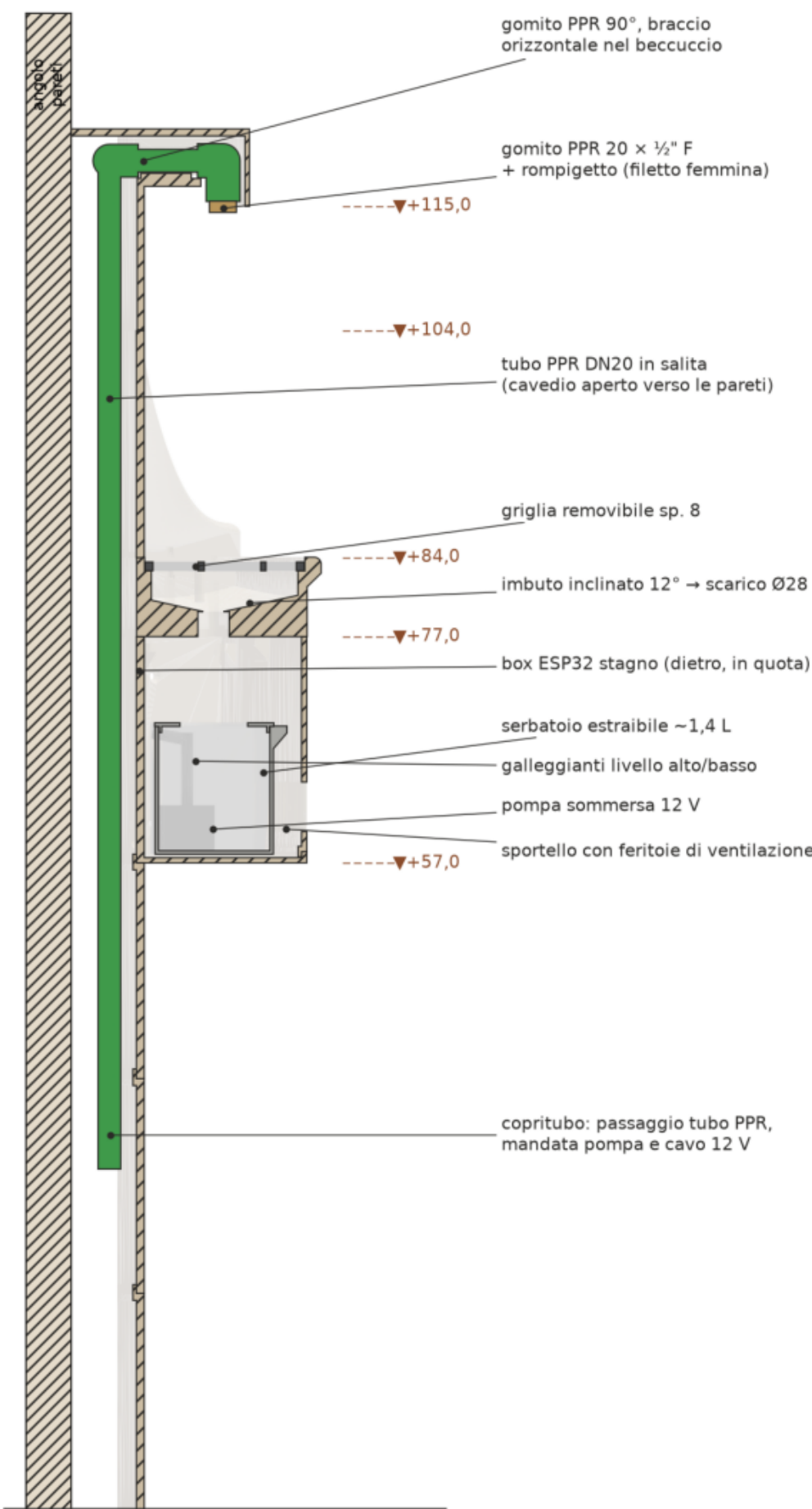
4 · Sezione con tubo PPR e vano tecnico
