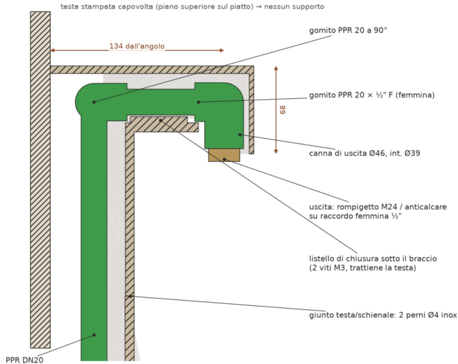
6 · Dettaglio beccuccio
