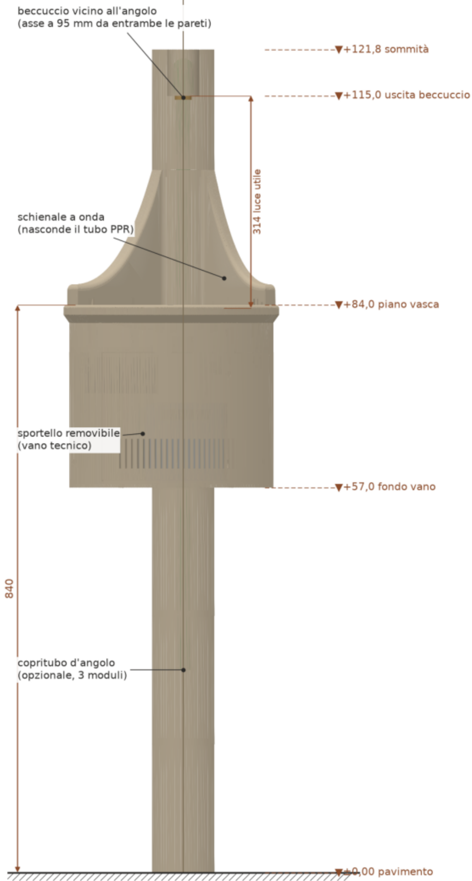
3 · Prospetto frontale
