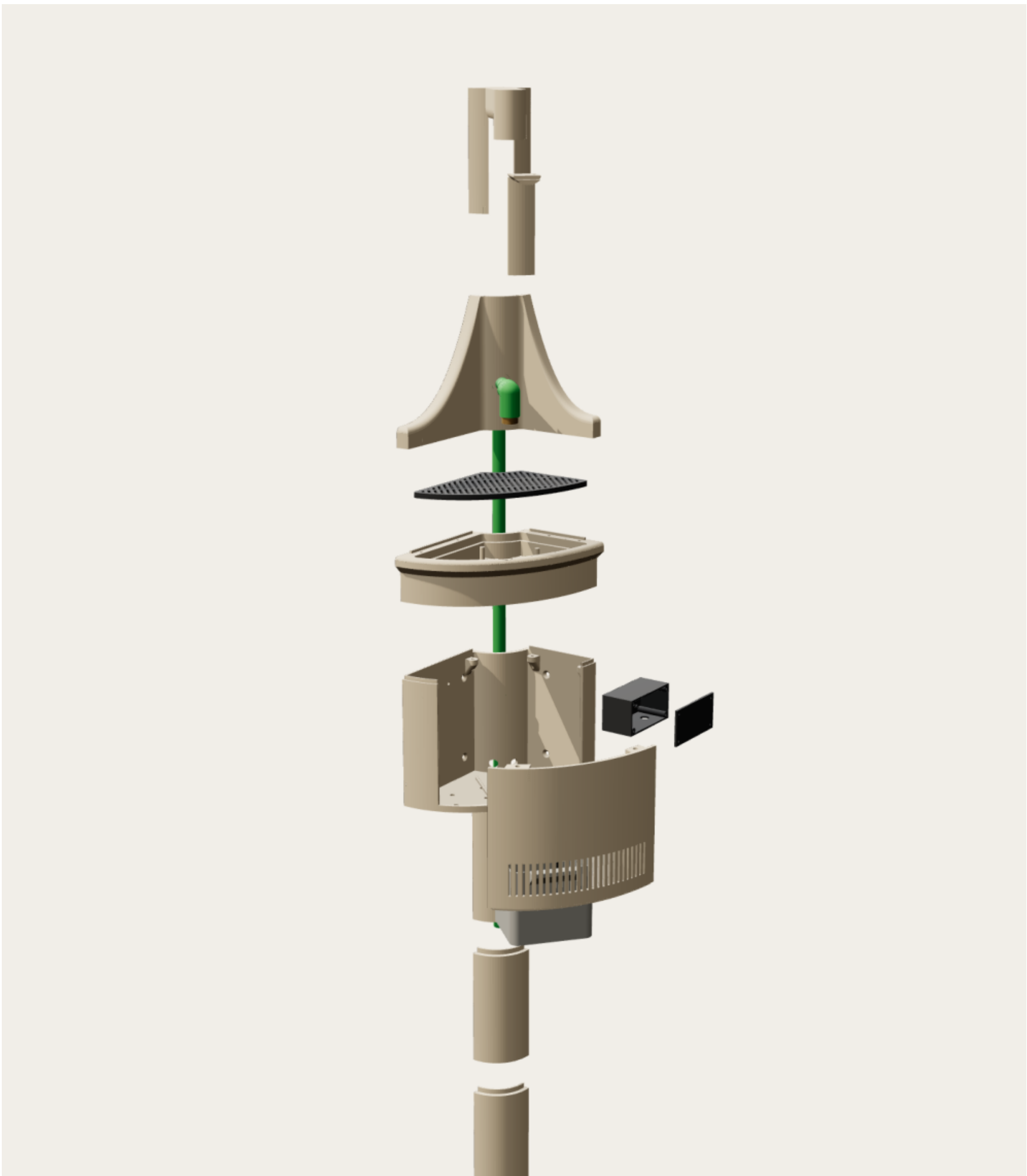
5 · Esploso
