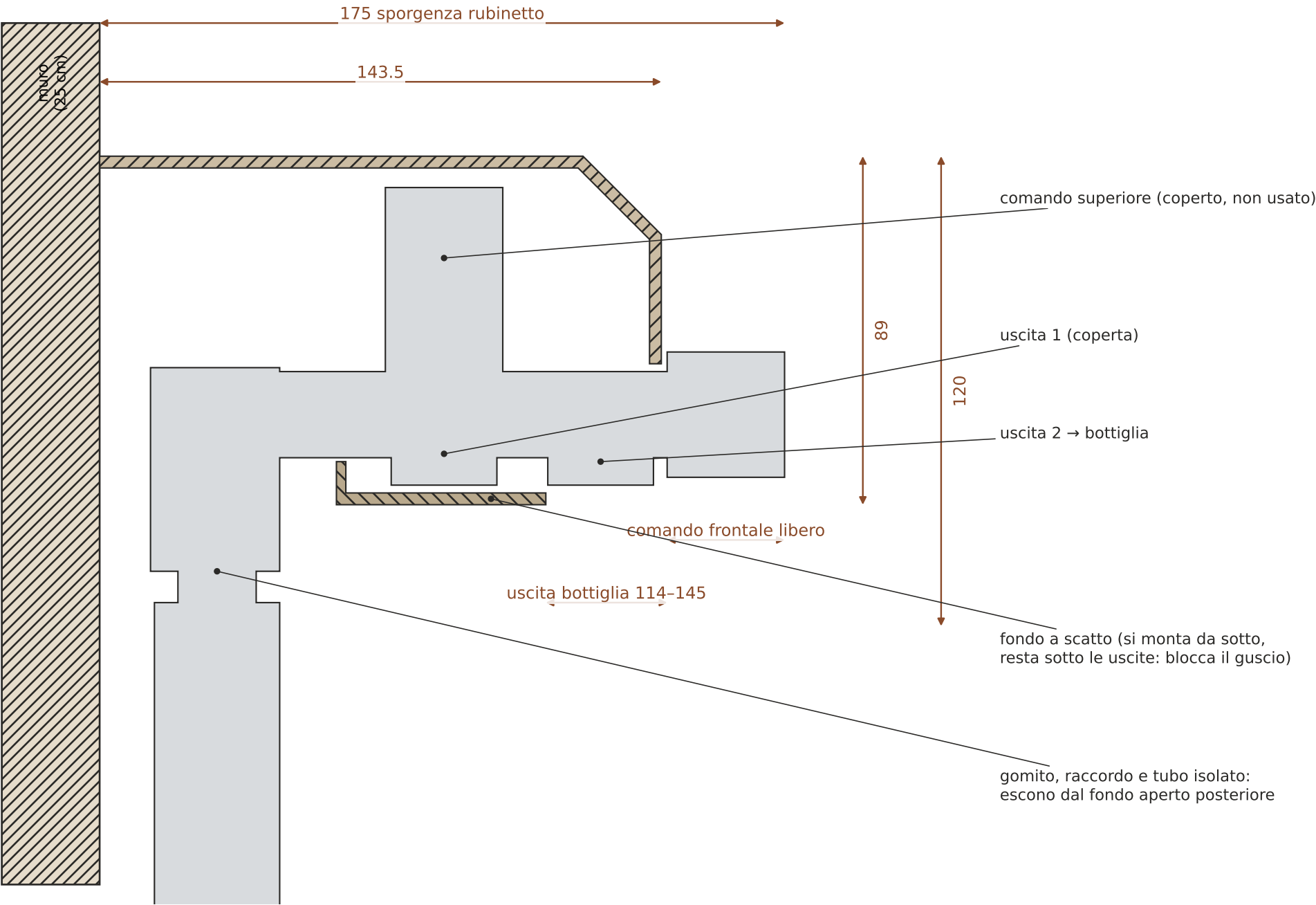
SEZIONE SULL'ASSE DEL RUBINETTO
