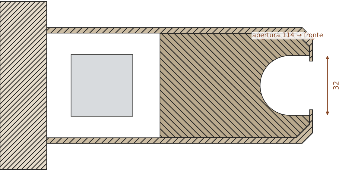
SEZIONE ORIZZONTALE AL FONDO
