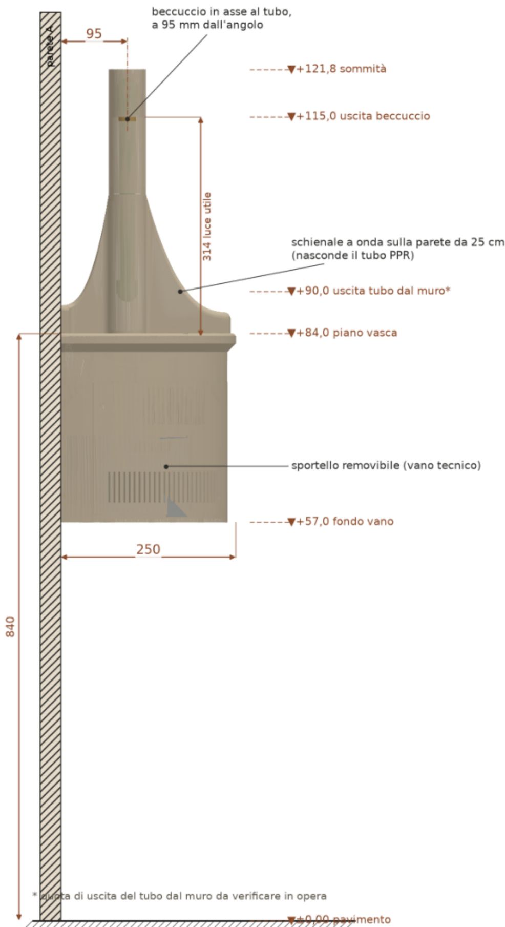
3 · Prospetto frontale
