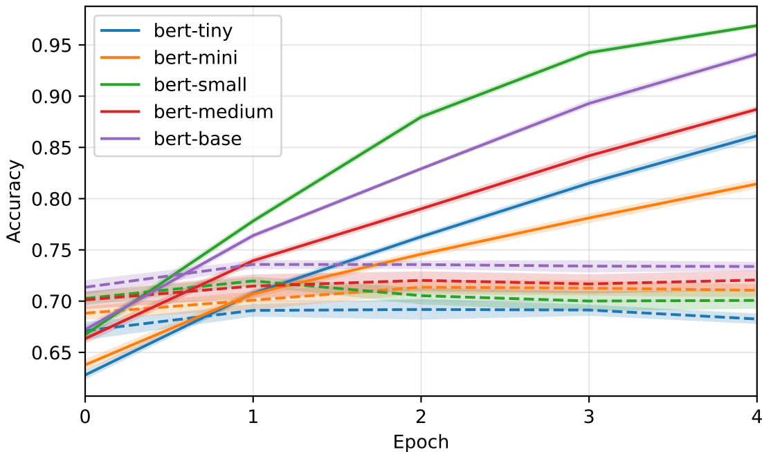
FigLang Dataset
