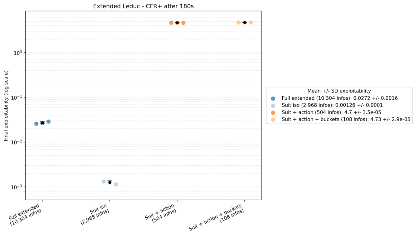
Фигура 4: Extended Ледюк CFR+ abstraction results
