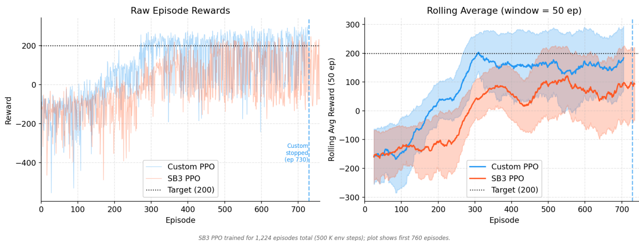
Фигура 2: PPO comparison - Custom vs SB3
