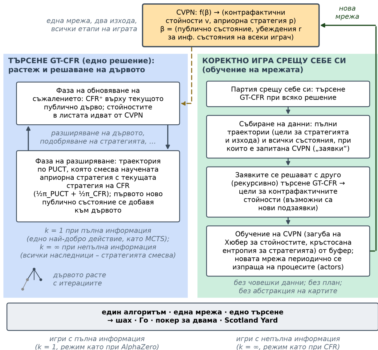
Фигура 28: Student of Games: цикълът на търсене GT-CFR (вляво) и цикълът на коректна игра срещу себе си, който го хранва (вдясно), използват една и съща CVPN; долната лента обобщава обединяването на игрите с пълна и с непълна информация.
