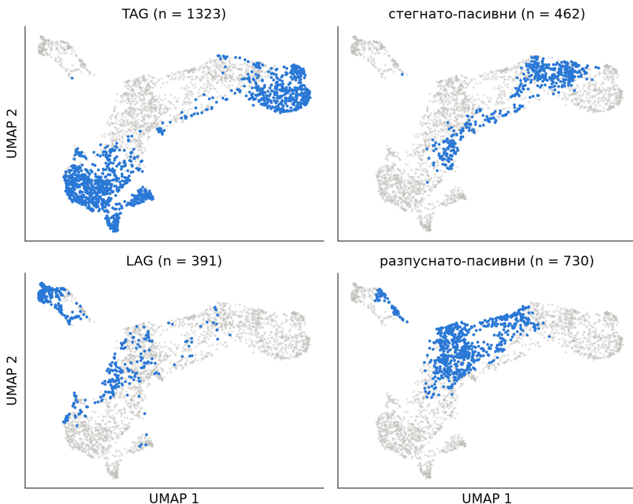
Фигура 82: UMAP проекция на вгражданията player2vec на 2 906-те редовни играчи в iPoker (начално число 0), по един панел за всеки квадрант VPIP × PFR, открит в синьо върху всички играчи в сиво. Квадрантите заемат различни области на картата, като разпуснато-агресивните играчи са отчасти в отделен остров.
