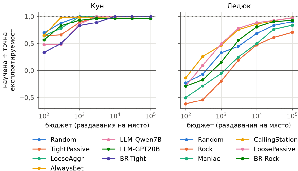
Фигура 8: Експлоатируемост, открита от научен най-добър отговор (таблично управление по метода Монте Карло, \varepsilon = 0,1 ), разделена на точната експлоатируемост, при нарастване на бюджета за обучение; средно по 3 начални числа и двете места.
