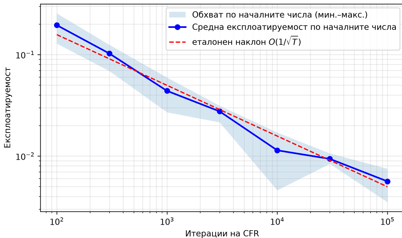
Фигура 2: Експлоатируемост на средната стратегия спрямо броя на итерациите в двулогаритмичен мащаб, средно за пет начални числа; оцветената ивица показва обхвата между тях. Измерените точки следват приблизително еталонния наклон O(1/\sqrt{T}) (прекъснатата линия), което съответства на теоретичната граница.
