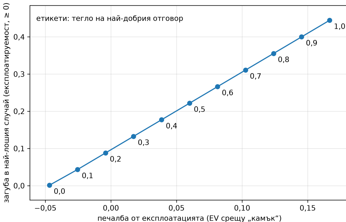
Фигура 27: Наивното смесване на равновесието на Наш с най-добрия отговор очертава плавна граница между експлоатация и безопасност в Кун: всяка стъпка към по-голяма печалба струва почти пропорционално нарастване на собствената загуба в най-лошия случай.
