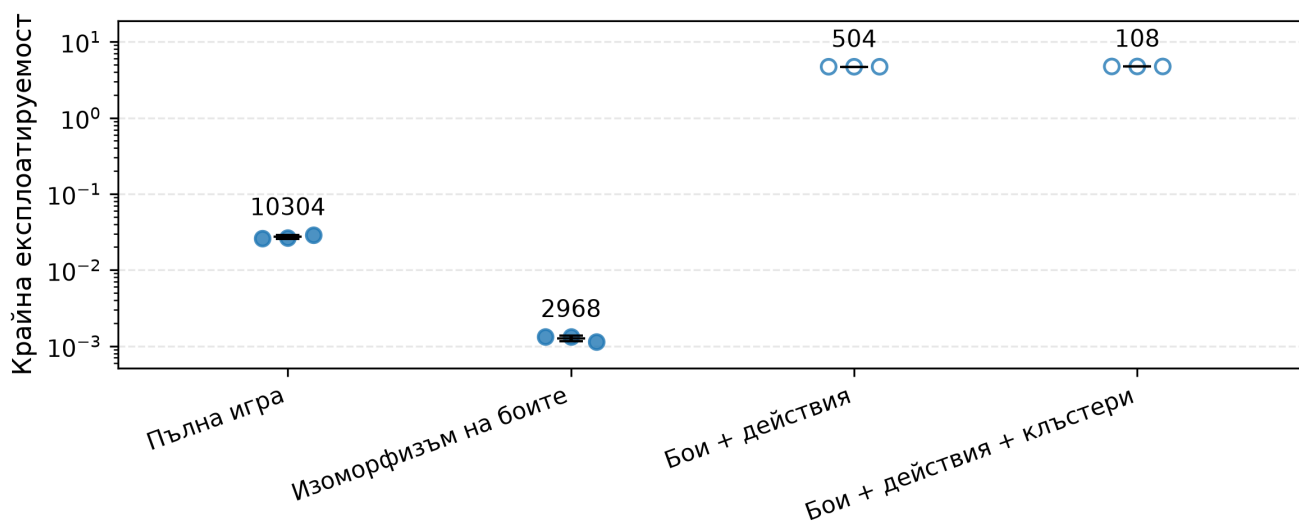
Фигура 4: Разширен Ледюк: крайна експлоатируемост след 180 s CFR+ за пълната игра, изоморфизма на боите и комбинираните абстракции; числото над всяка група е броят информационни множества. Незапълнените маркери отбелязват конфигурациите с абстракция на действията (вж. текста).
