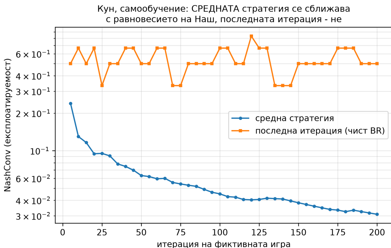
Фигура 9: Самообучение в Кун: експлоатируемостта (NashConv) на средната стратегия постепенно спада към нула, докато тази на последната итерация продължава да се колебае. Затова самообучението и PSRO разчитат на осредняване по популацията, а не на последната стратегия.
