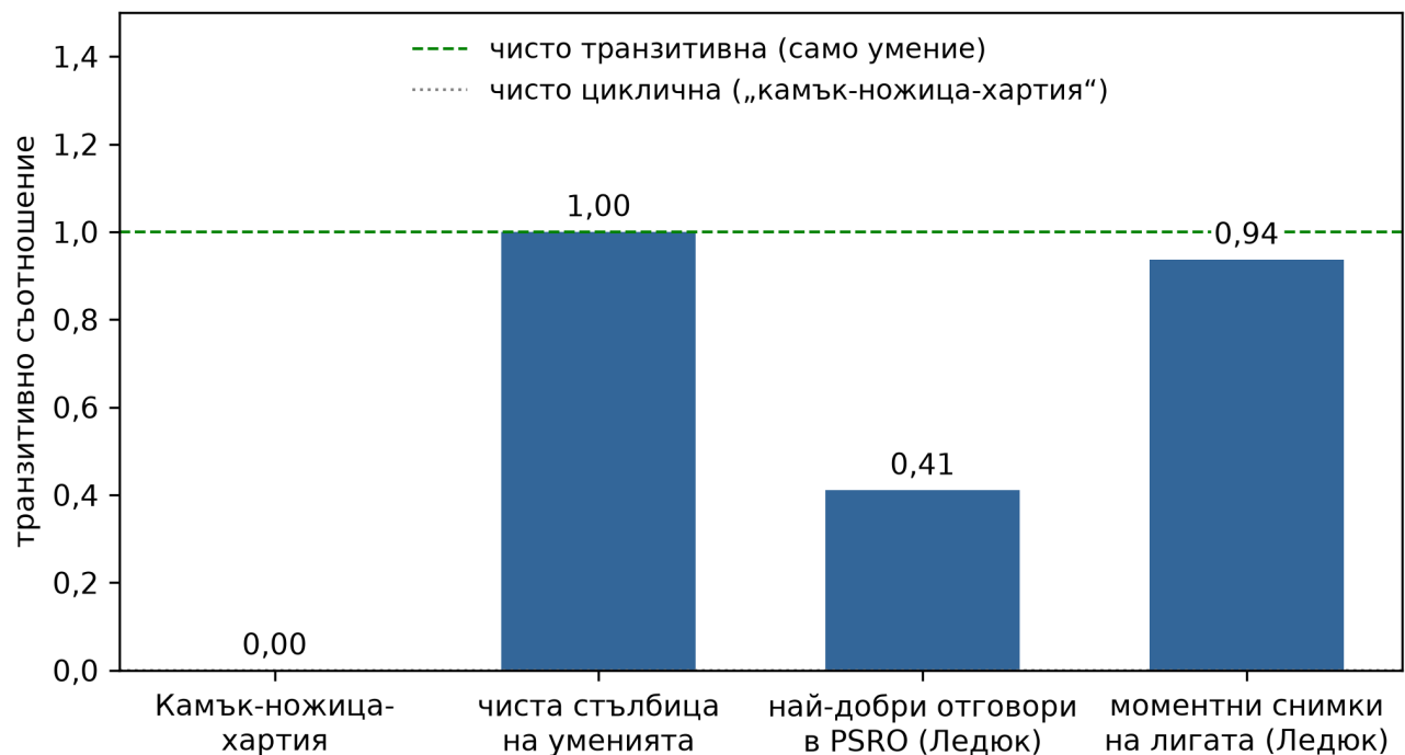
Фигура 4: Транзитивно съотношение на четири популации: „камък-ножица-хартя“ (0,0, чисто циклична), чиста стълбица на уменията (1,0), мета-играта на най-добрите отговори в PSRO за Ледюк (~0,41-0,46, предимно циклична) и мета-играта на моментните снимки на лигата (~0,94-0,98, предимно транзитивна). Една и съща игра има противоположна структура в зависимост от това как е изградена популацията.
