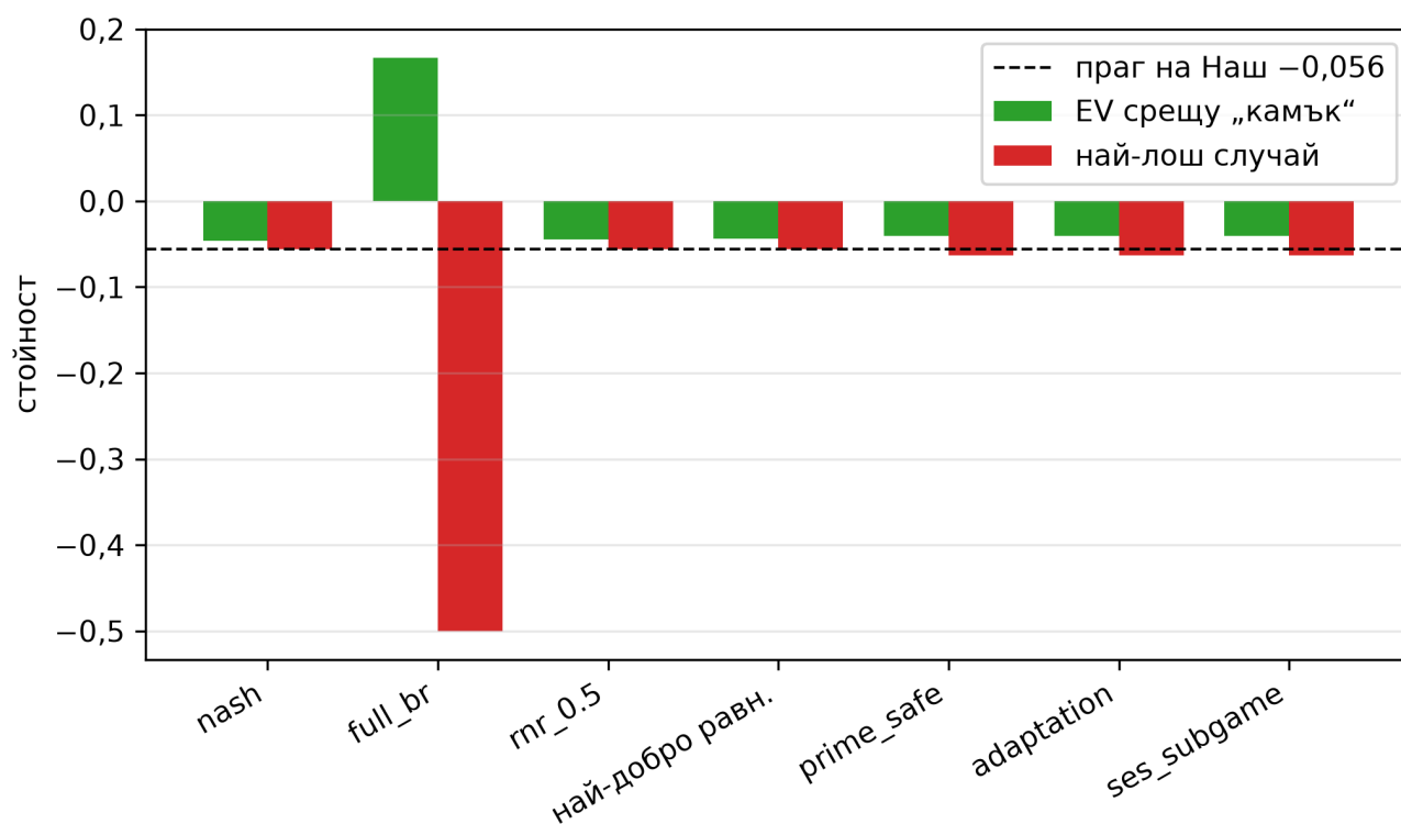
Фигура 4: Методите срещу „камък“ в Кун: в зелено е очакваната стойност срещу противника, в червено - стойността в най-лошия случай, а пунктирът е прагът на Наш. Само при пълния най-добър отговор стойността в най-лошия случай (червено) пада до -0.5 , далеч под прага; всички строго обосновани методи остават близо до прага и печелят колкото равновесието или малко повече.
