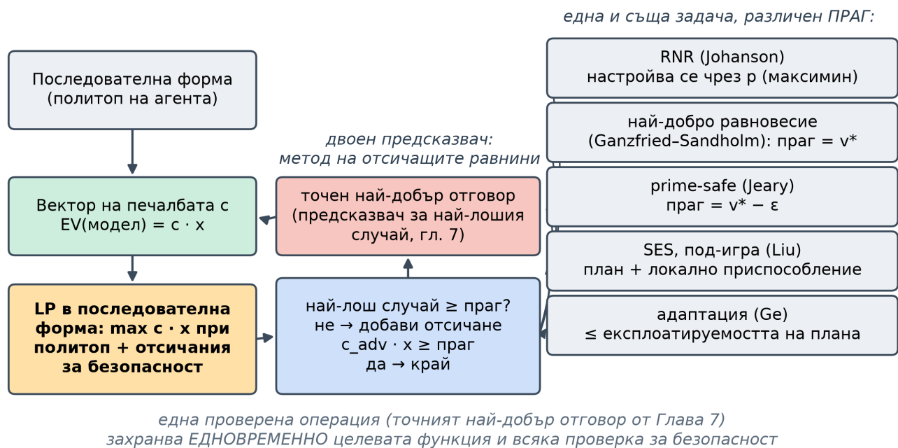
Фигура 39: Една LP-задача, пет прага: точният най-добър отговор служи като предсказвач за най-лошия случай и добавя отсичащи ограничения, докато прагът не бъде спасен; RNR, най-доброто равновесие, prime-safe, SES и адаптацията се различават единствено по прага.
