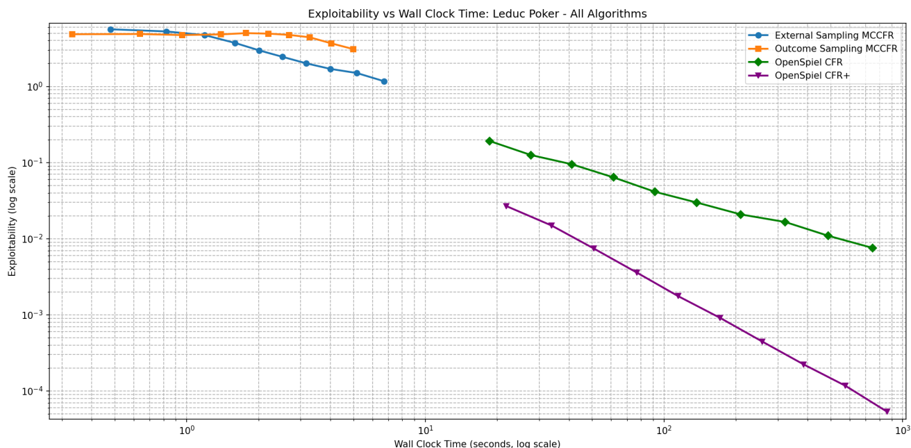
Фигура 7: Ледюк Poker - Exploitability vs Wall-Clock Time
