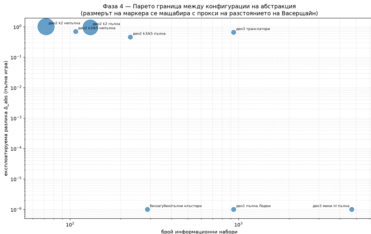
Фигура 4: Abstraction Pareto frontier
