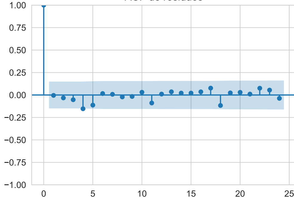
ACF de residuos
