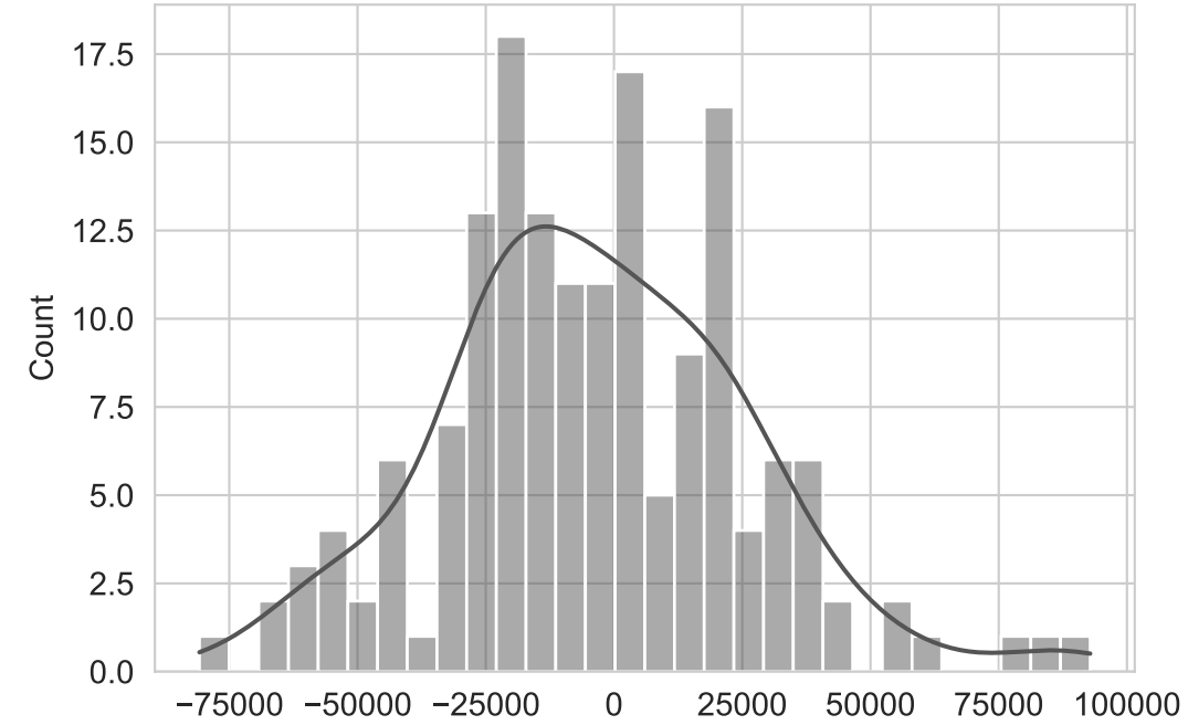
Distribucion de residuos
