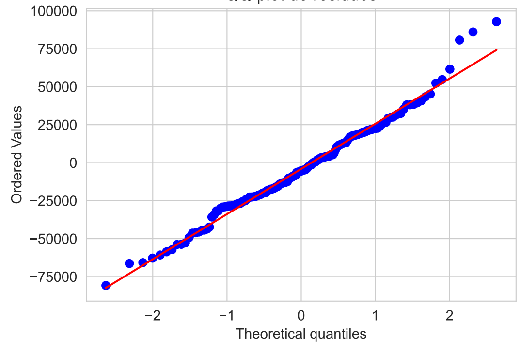
QQ-plot de residuos
