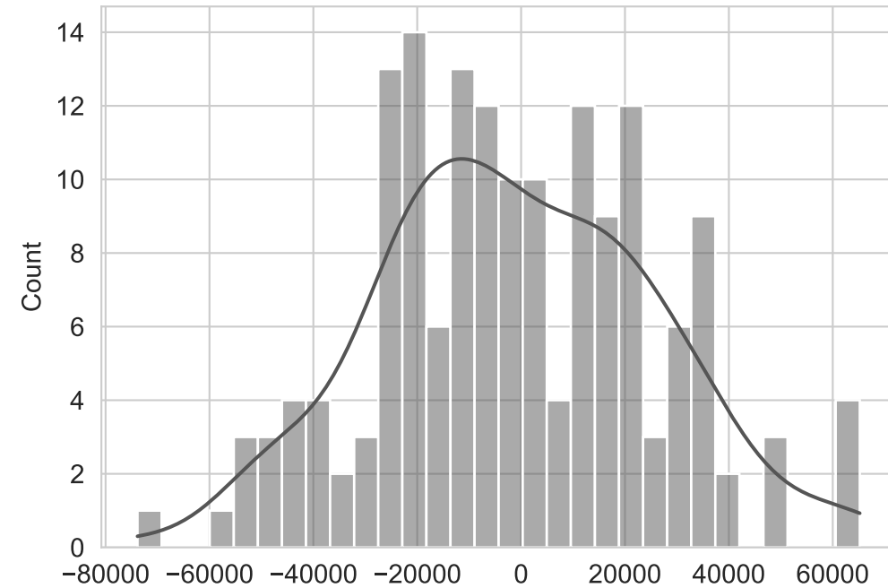
Distribucion de residuos
