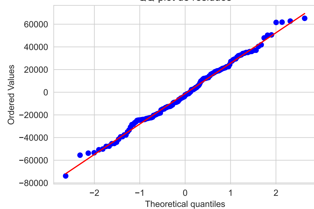
QQ-plot de residuos
