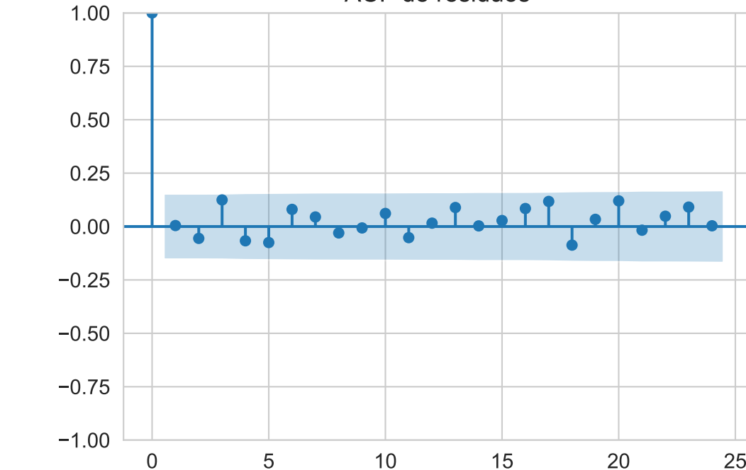
ACF de residuos
