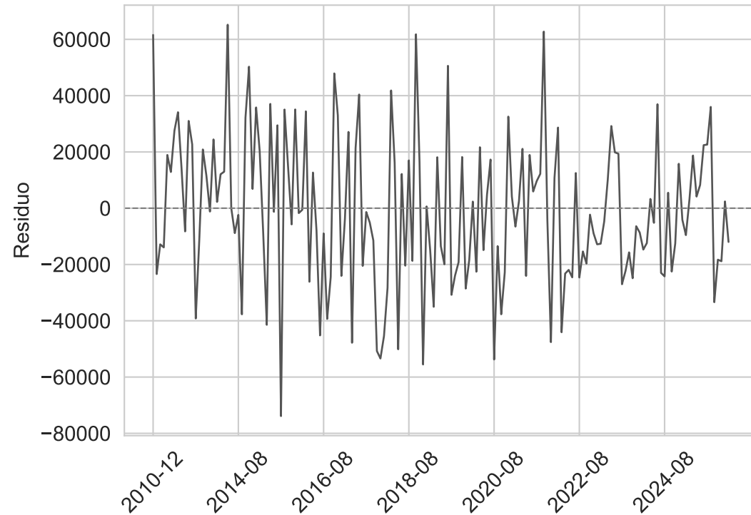
Residuos en el tiempo
