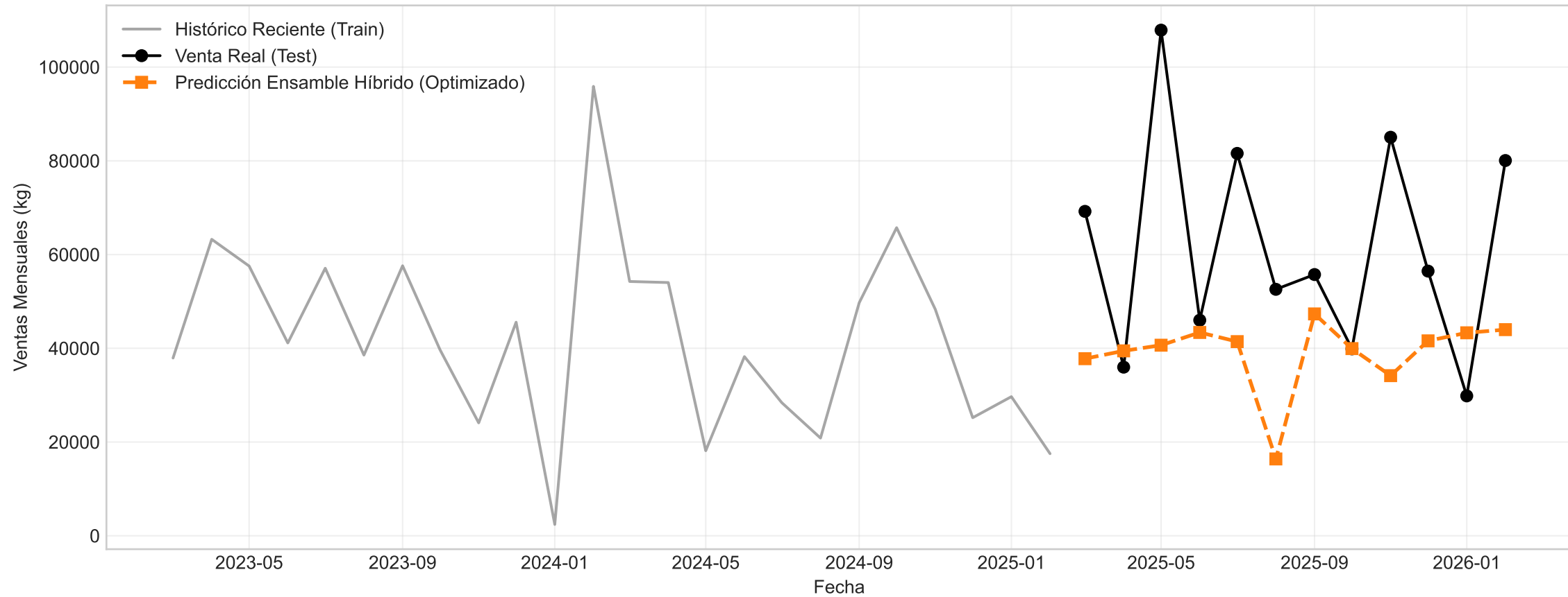
Familia 124: Ensemble Óptimo RF + LightGBM (Sin Lag)
