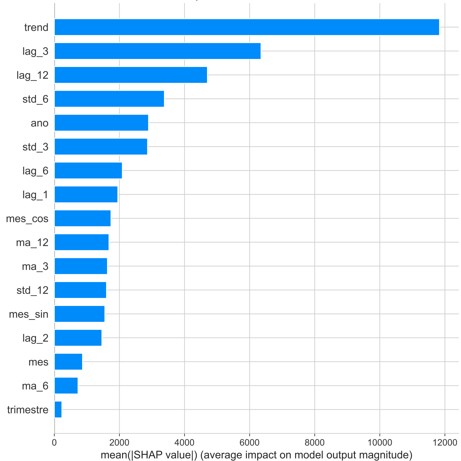
SHAP Importancia media — XGBoost 233
