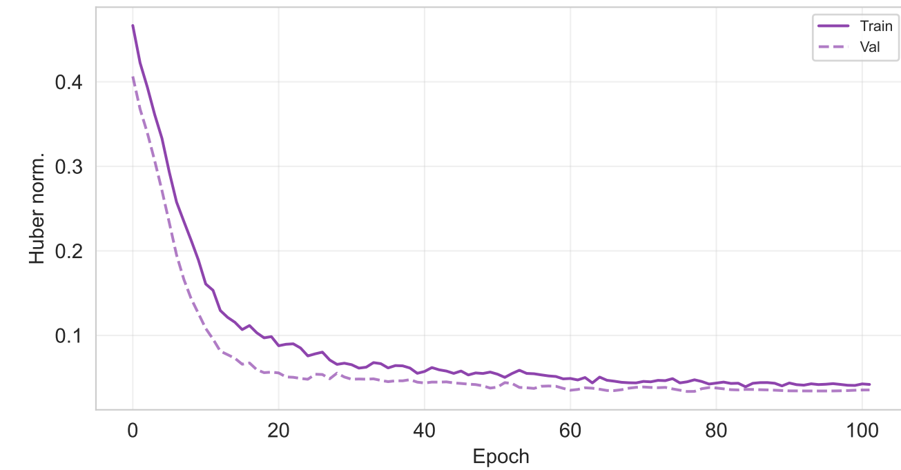
GRU — 233 (102 epochs)
