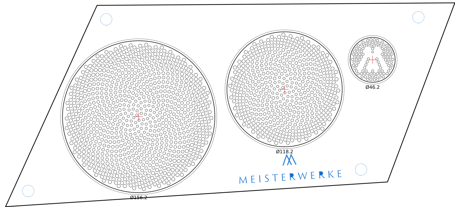
Ansicht von vorn (linke Bootsseite) M 1:2
