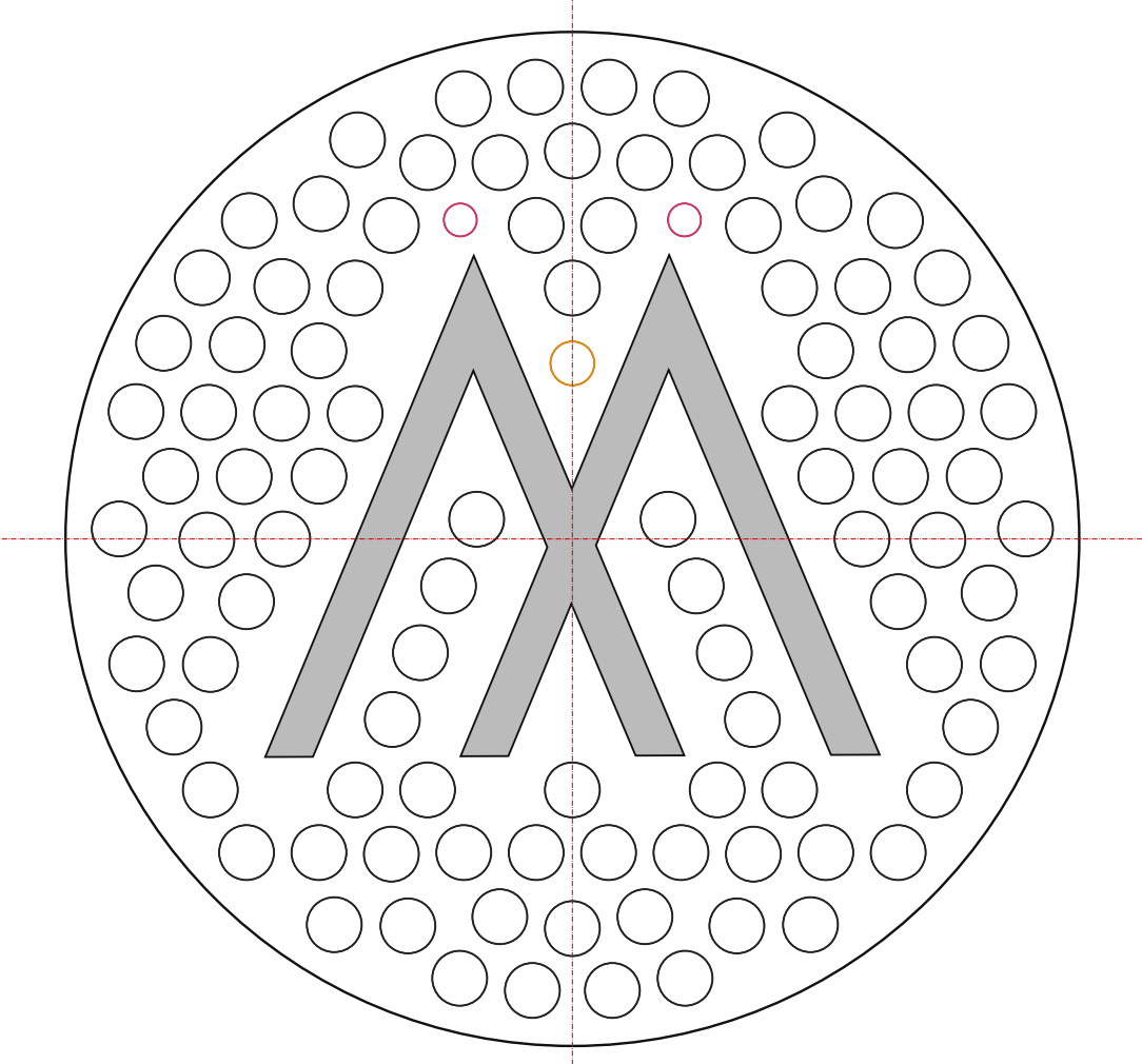
Detail Hochtöner-Feld Ø46,2 M 3:1
