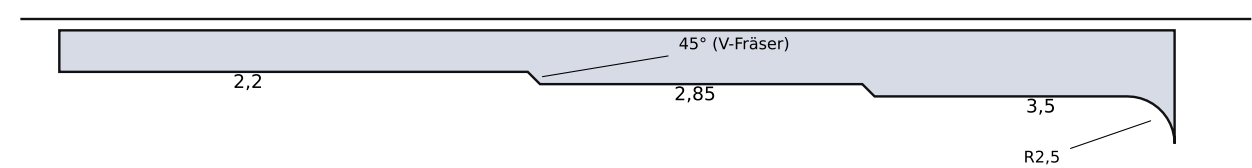
Schnitt durch Feld Ø118,2 (Haut) M 2:1
