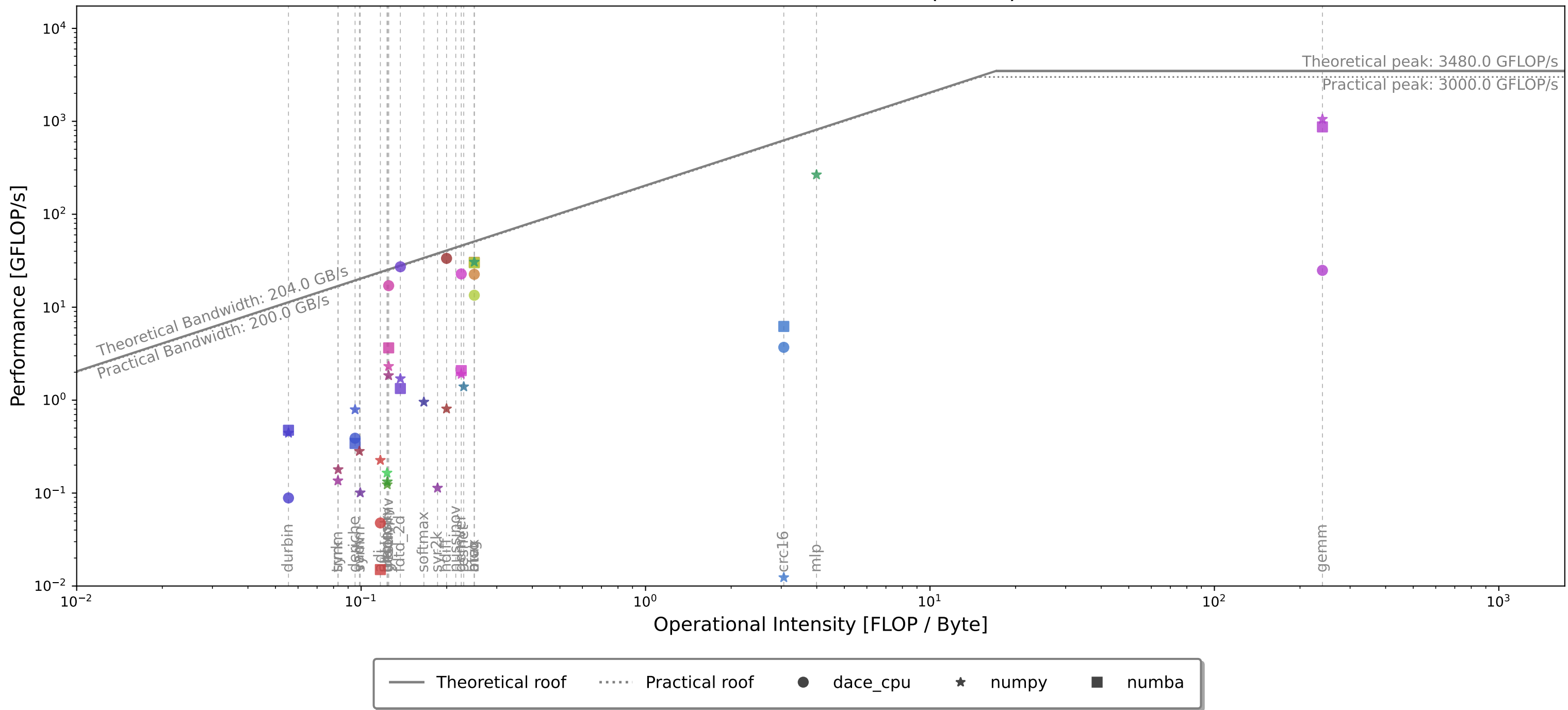
CPU Roofline EPYC 7742 (Rome)
