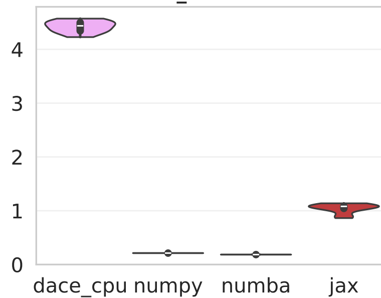
bicg
