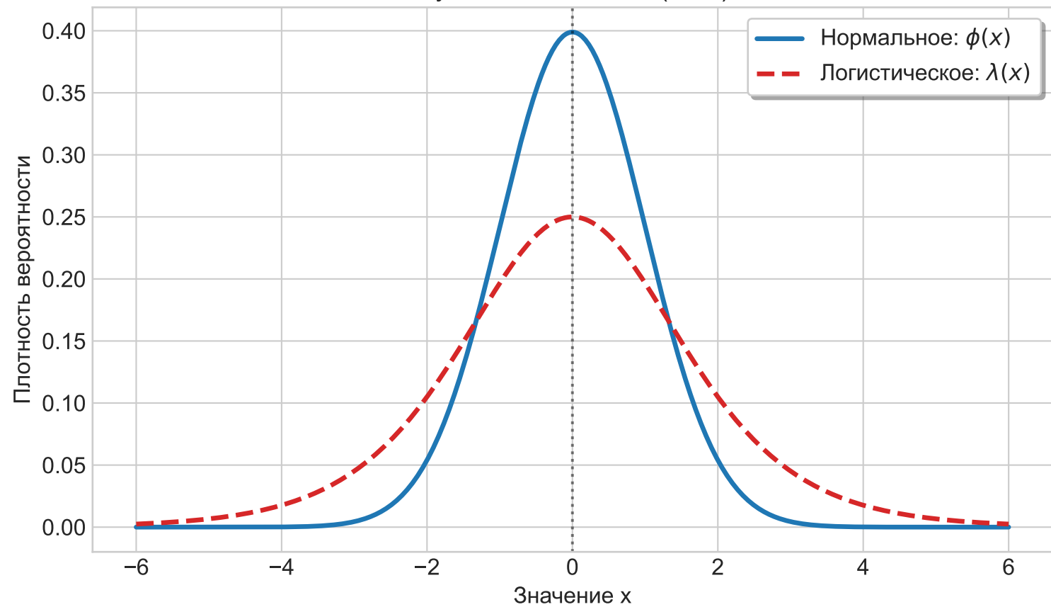
Функция плотности (PDF)
