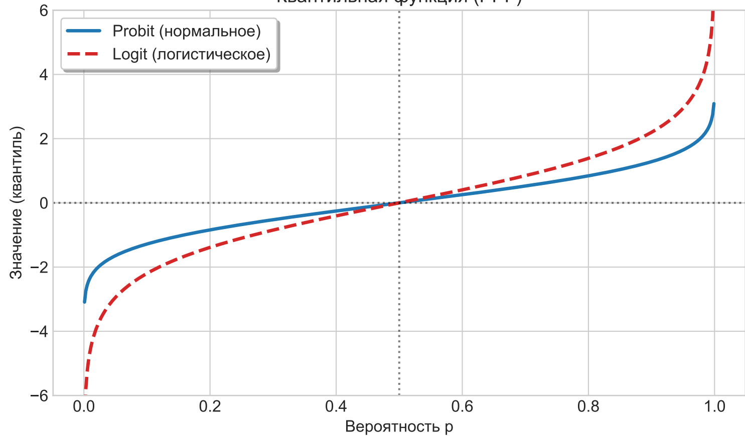
Квантильная функция (PPF)
