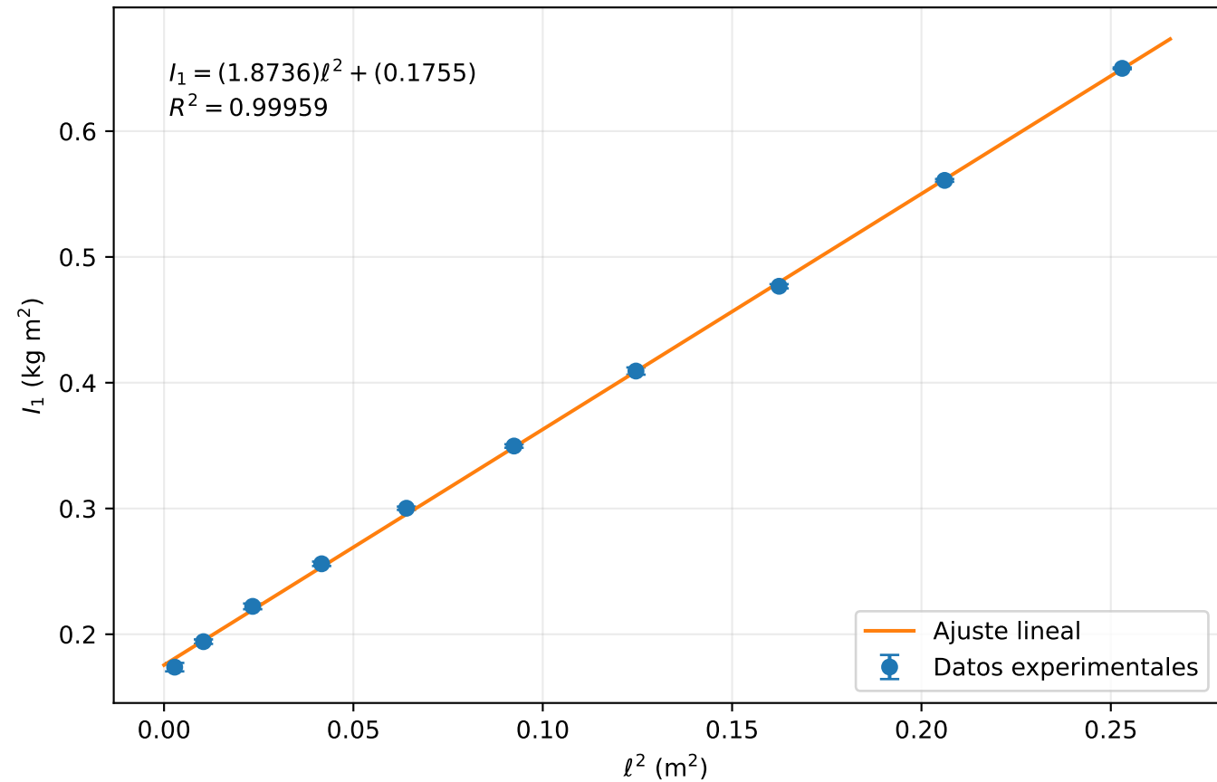
Momento de inercia en función de \ell^2
