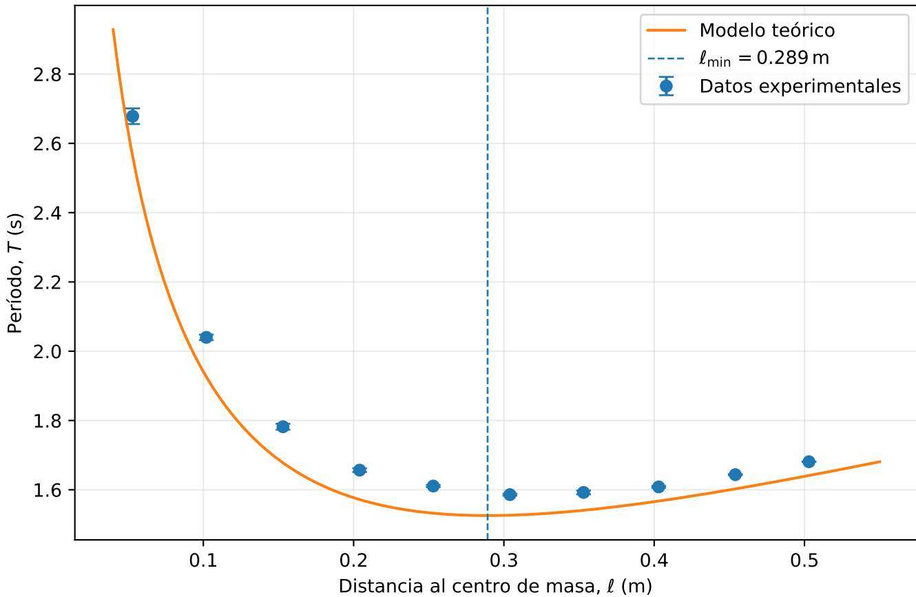
Período de oscilación en función de \ell
