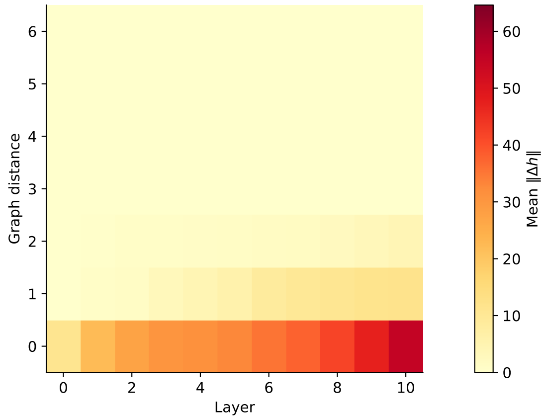
ZINC — VNode (GRIT)
