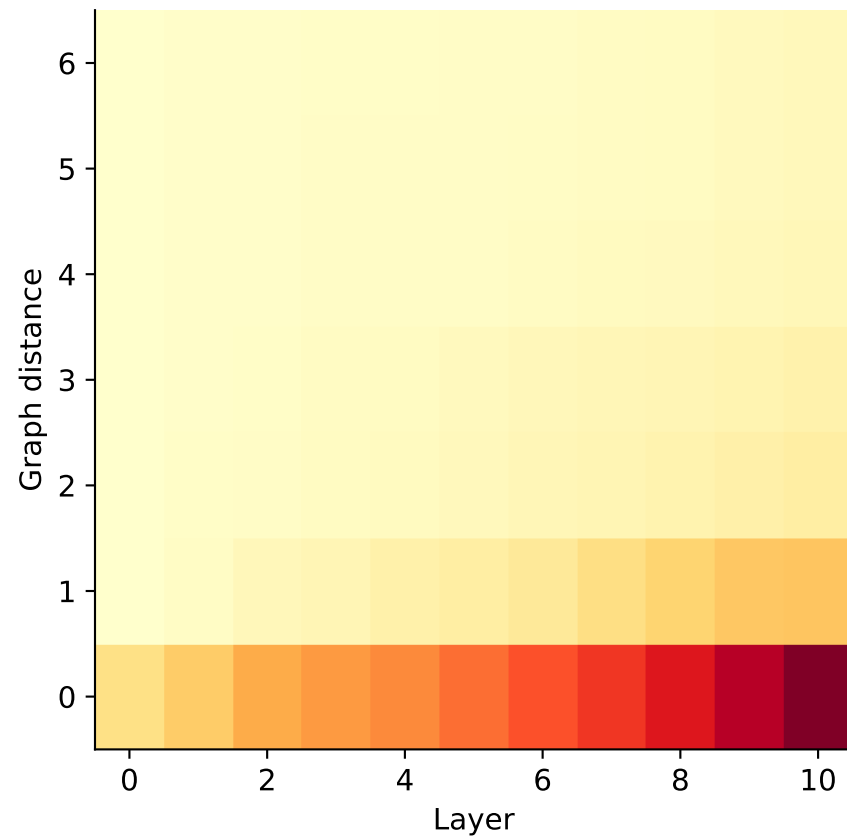
ZINC — No VNode (GRIT)
