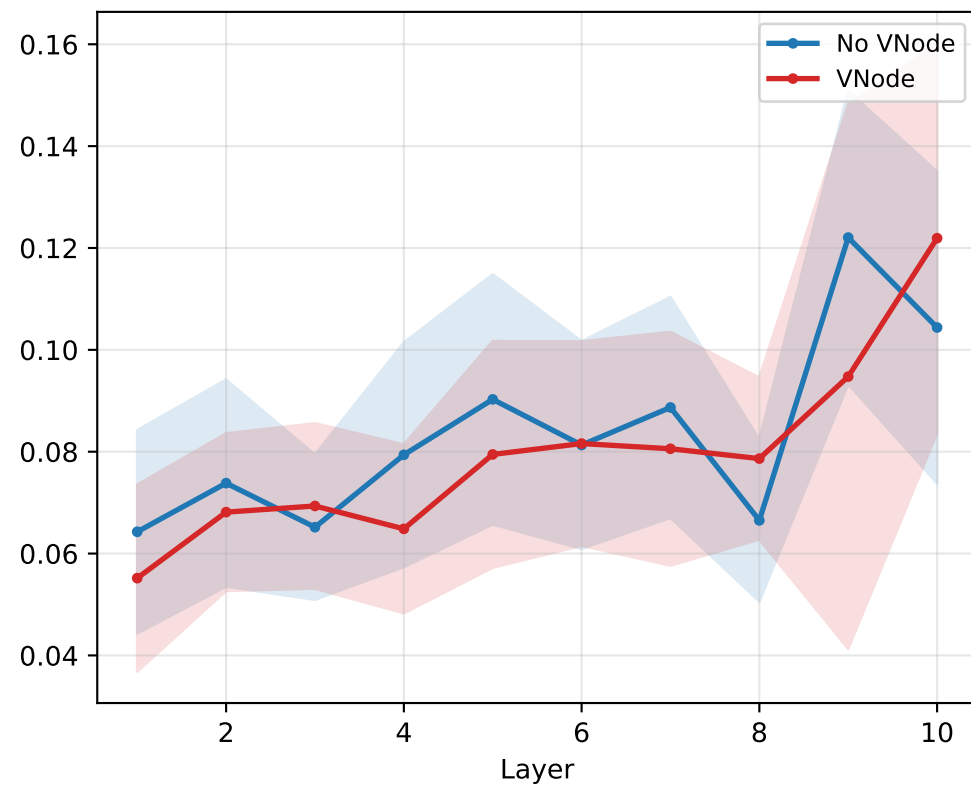
Anisotropy p_1
