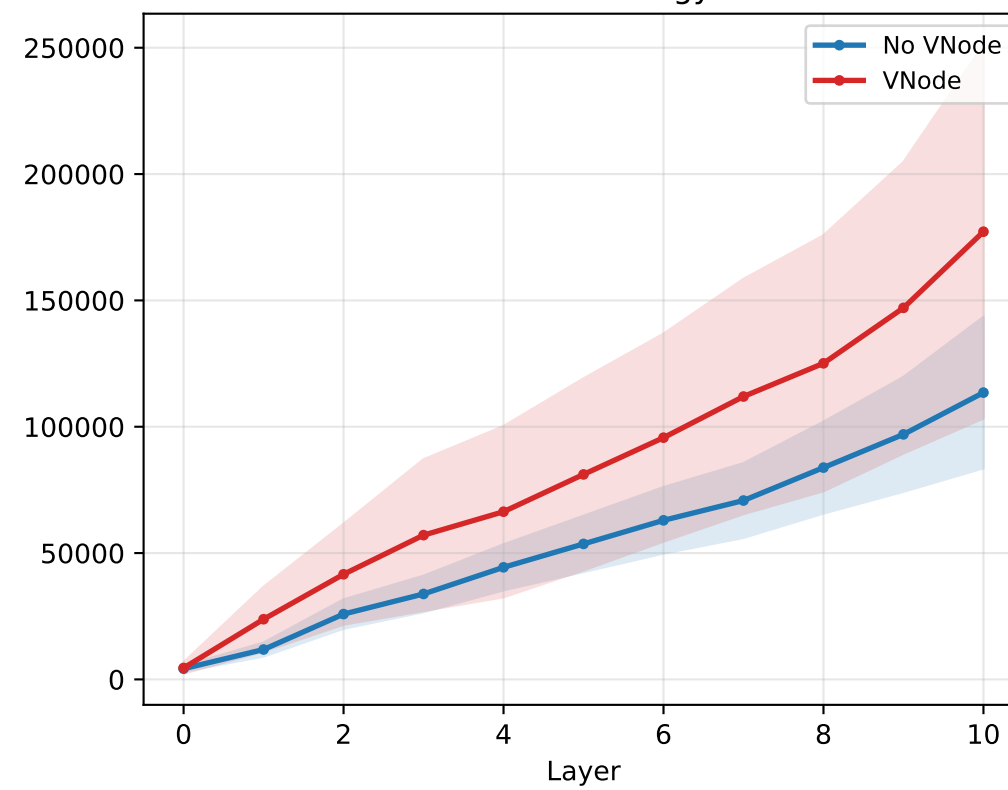
Dirichlet Energy
