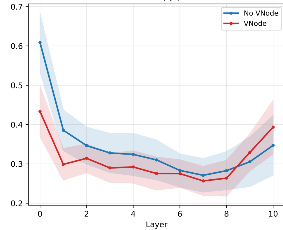
Anisotropy p_1
