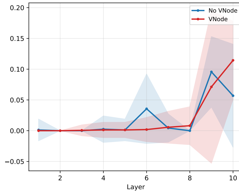
Dirichlet Energy
