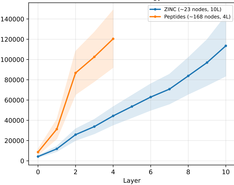
Dirichlet Energy
