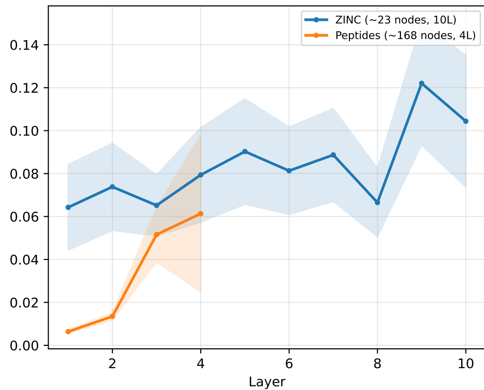
Anisotropy p_1
