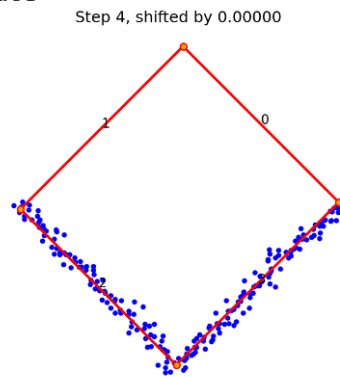
(d) \alpha = 0.20
