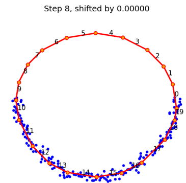
(d) \alpha = 0.20
