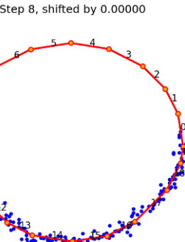
(d) \alpha = 0.20
